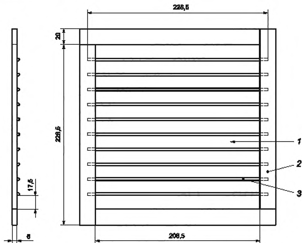
1 — направление воздушного потока в испытательной камере; 2 — латунь 20×6 мм; 3 — планка из нержавеющей стали (диаметр 1,6 мм)
