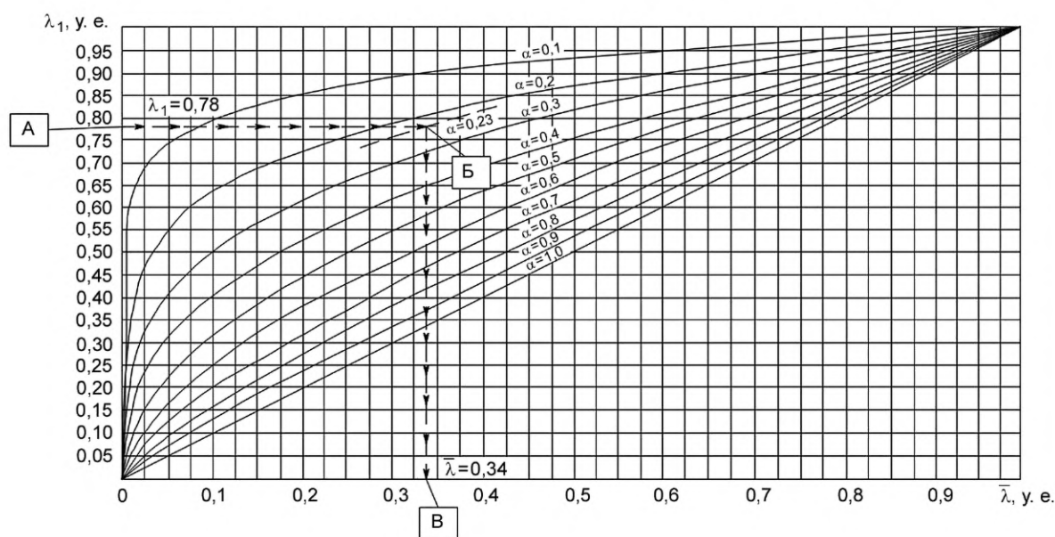
Рисунок A.5 — Номограмма к примеру определения значения показателя среднего размера \bar{\lambda} открытых капиллярных пор (при вспомогательном параметре \lambda_1 \leq 1 )
