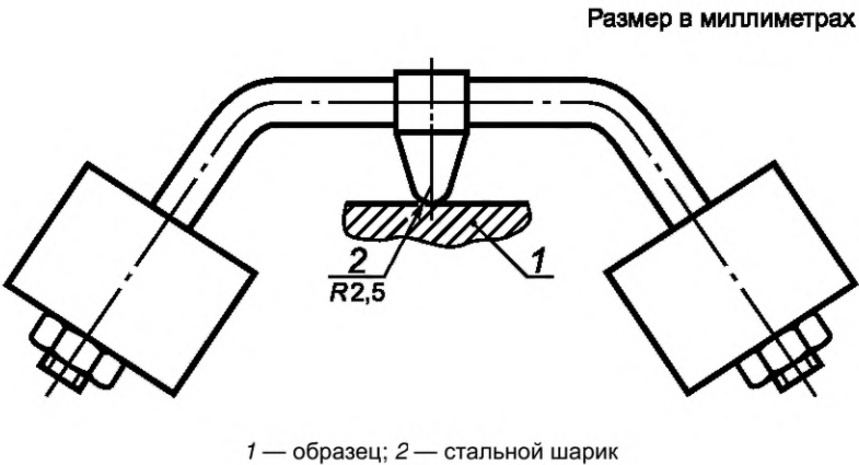
Рисунок 21 — Устройство для испытания давлением шарика (9.14.2)
