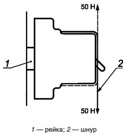
Рисунок 20 — Приложение усилия для испытания на механический удар АВДТ, монтируемых на рейке (9.13.2.2)
