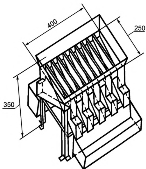
Рисунок 9 — Делитель Джонса
