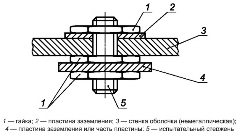
Рисунок 8 — Сборка испытательного образца для испытания целостности заземления
