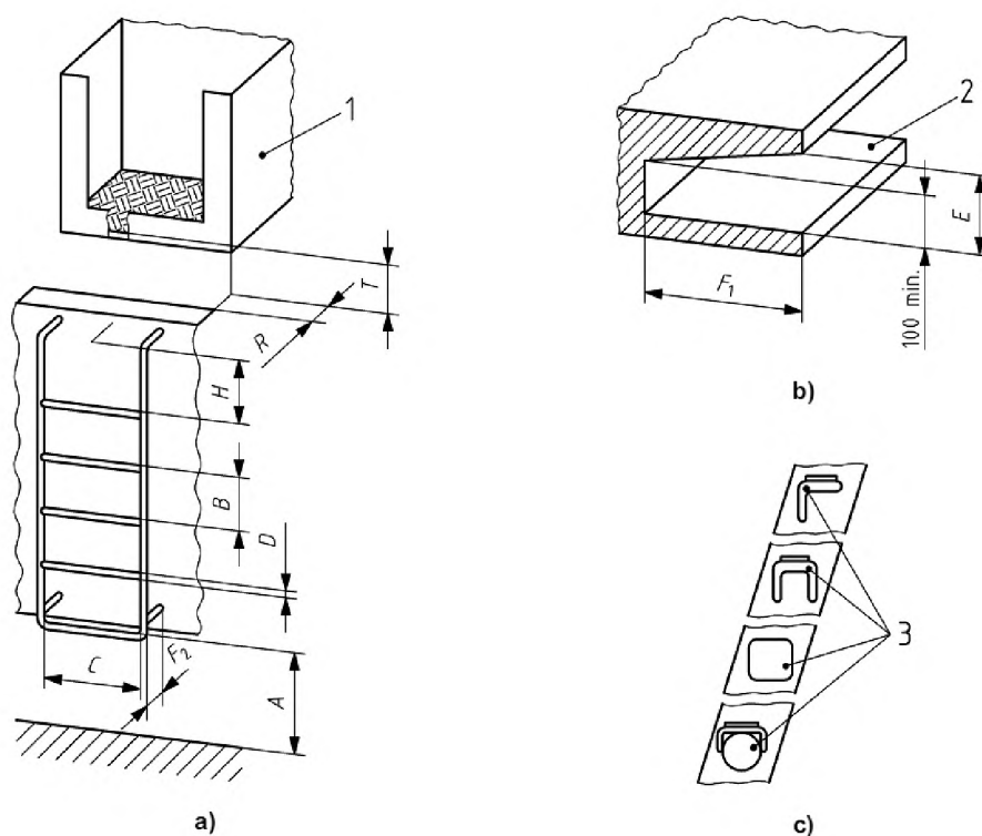
Рисунок G.1 — Размеры ступеней и лестниц
