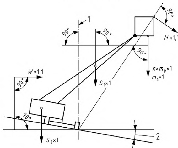
Рисунок 6 — Примеры 3a/3b и 4a/4b сочетаний максимальной опрокидывающей нагрузки и момента силы (см. таблицу 2)
