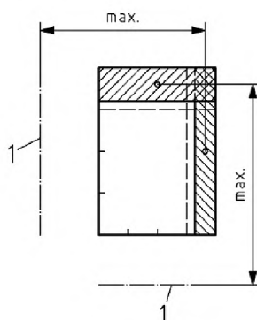
Рисунок 3 — Номинальная грузоподъемность (работающий персонал)
