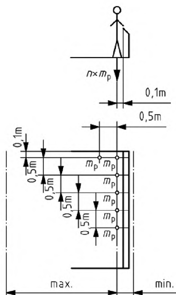
Рисунок 3 — Номинальная грузоподъемность (работающий персонал)
