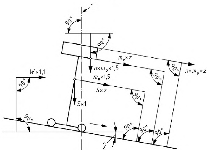
Рисунок 6 — Примеры 3a/3b и 4a/4b сочетаний максимальной опрокидывающей нагрузки и момента силы (см. таблицу 2)
