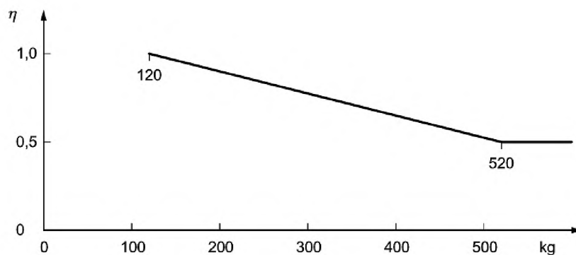
Рисунок 9 — Коэффициент спектральной нагрузки \eta
