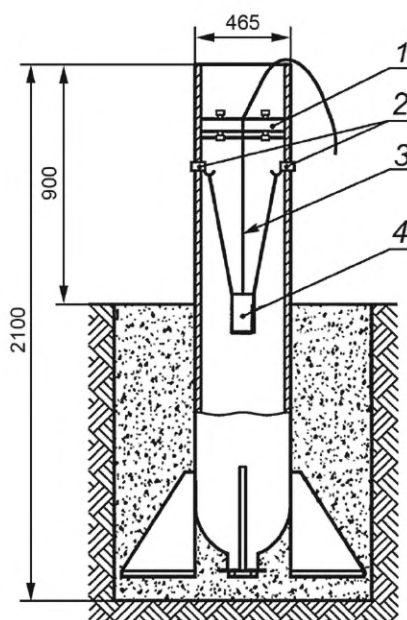
Рисунок 4б — Схема эффектомера 5 м 3
