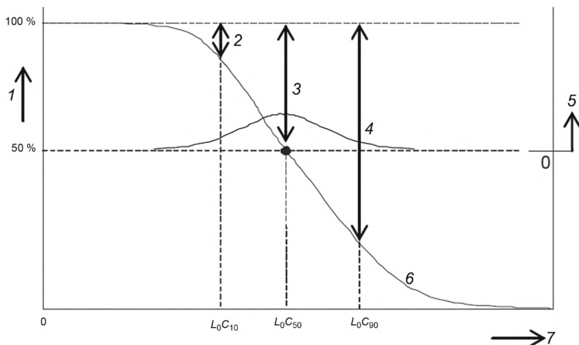
Рисунок Е.4 — Кривая надежности R_{резкое} для резкого падения светового потока
