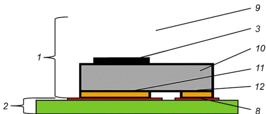
б) Поверхностный монтаж корпусированного СД без выводов
