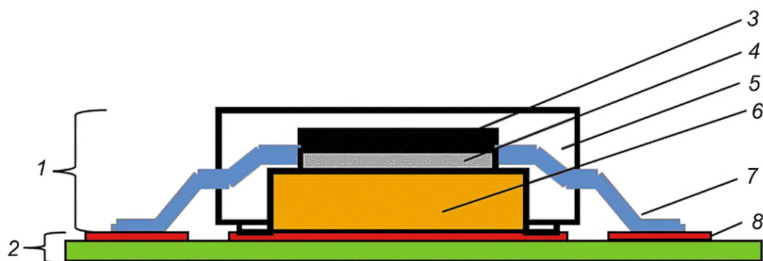
а) Поверхностный монтаж корпусированного СД с выводами
