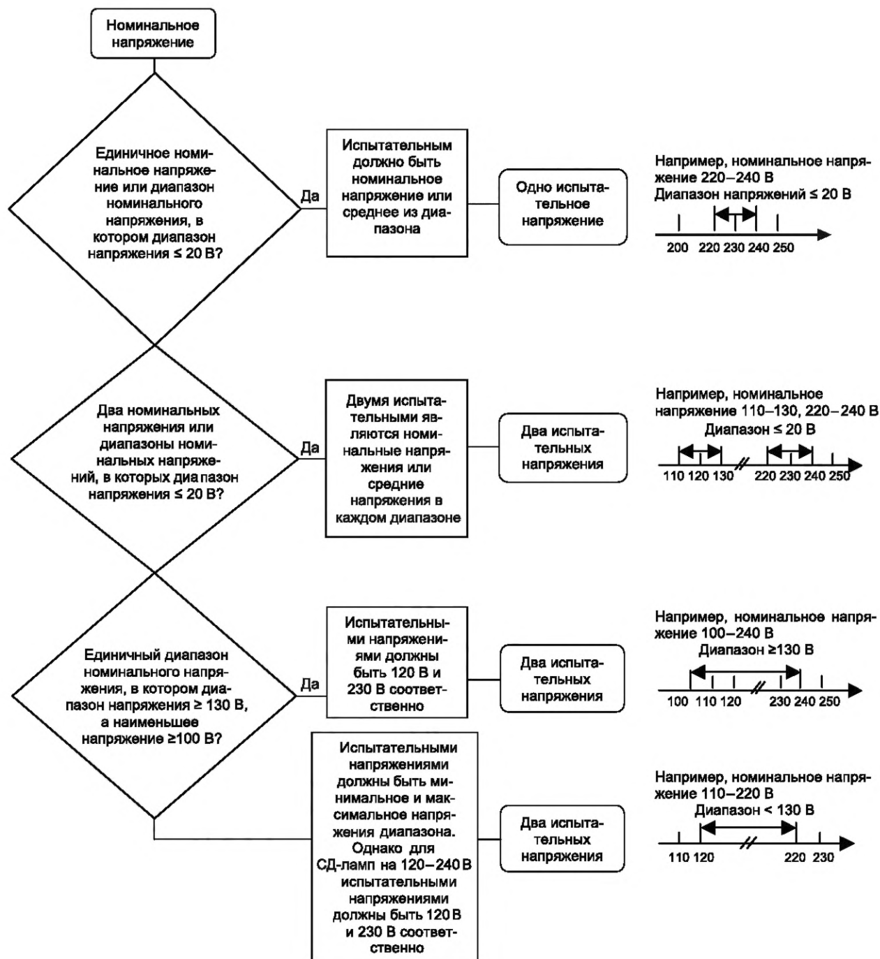
Рисунок А.1 — Зависимость номинального напряжения от испытательного
