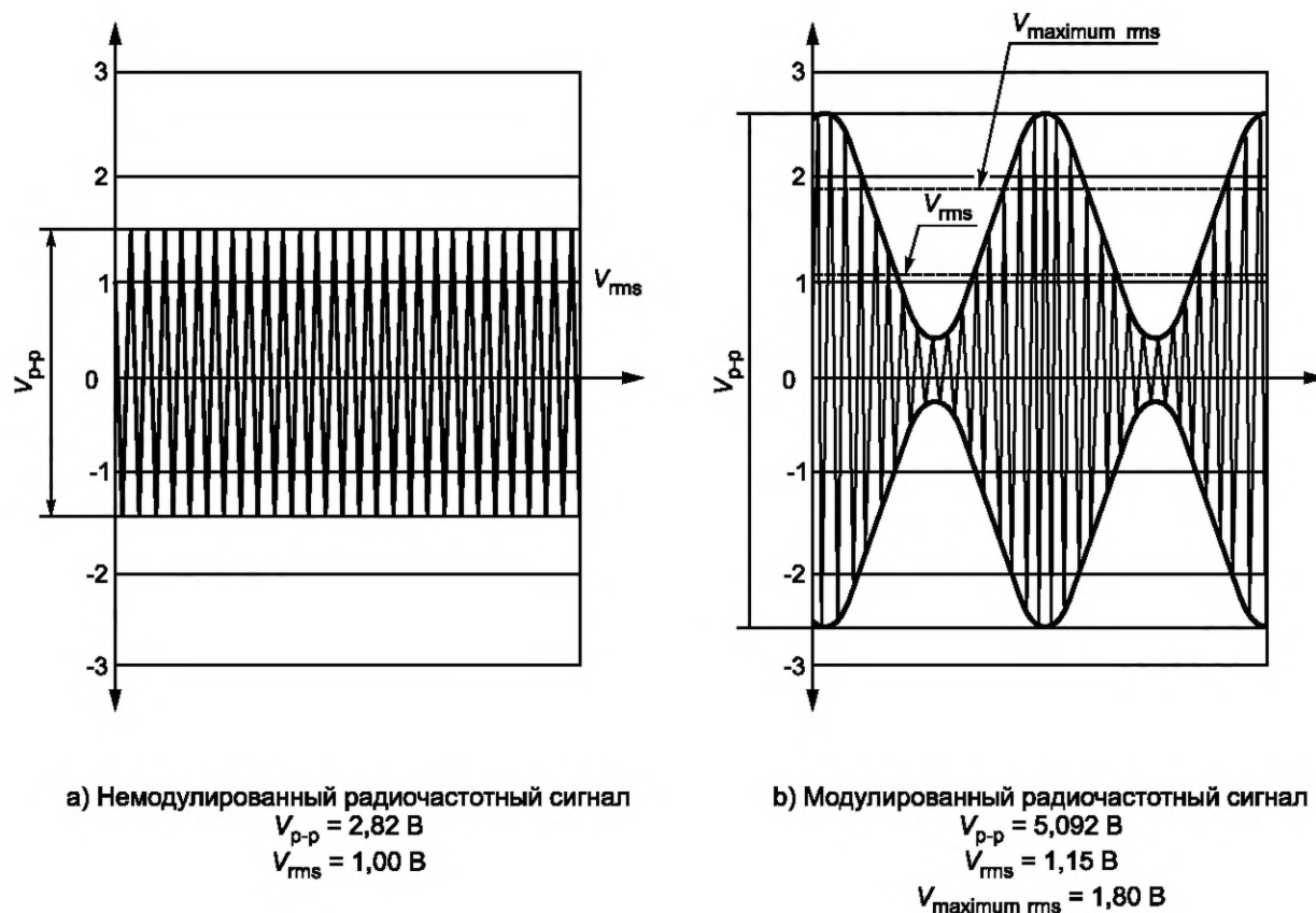
Рисунок 3 — Параметры амплитудно-модулированного (АМ) испытательного сигнала с глубиной модуляции 80 % и форма сигнала на выходе генератора сигналов
