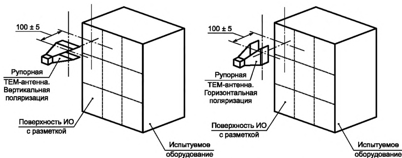
Рисунок 12 — Пример ориентации рупорной ТЕМ-антенны
