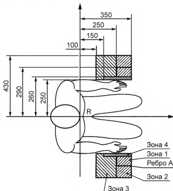
Рисунок 1 — Расположение органов управления в кабине
