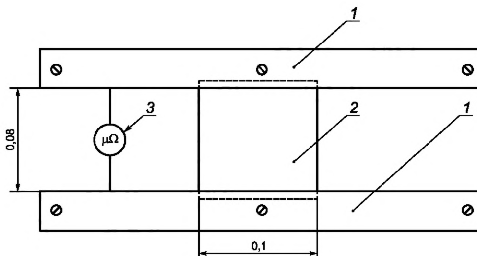
1 — медные пластины; 2 — испытуемый образец; 3 — микроомметр
