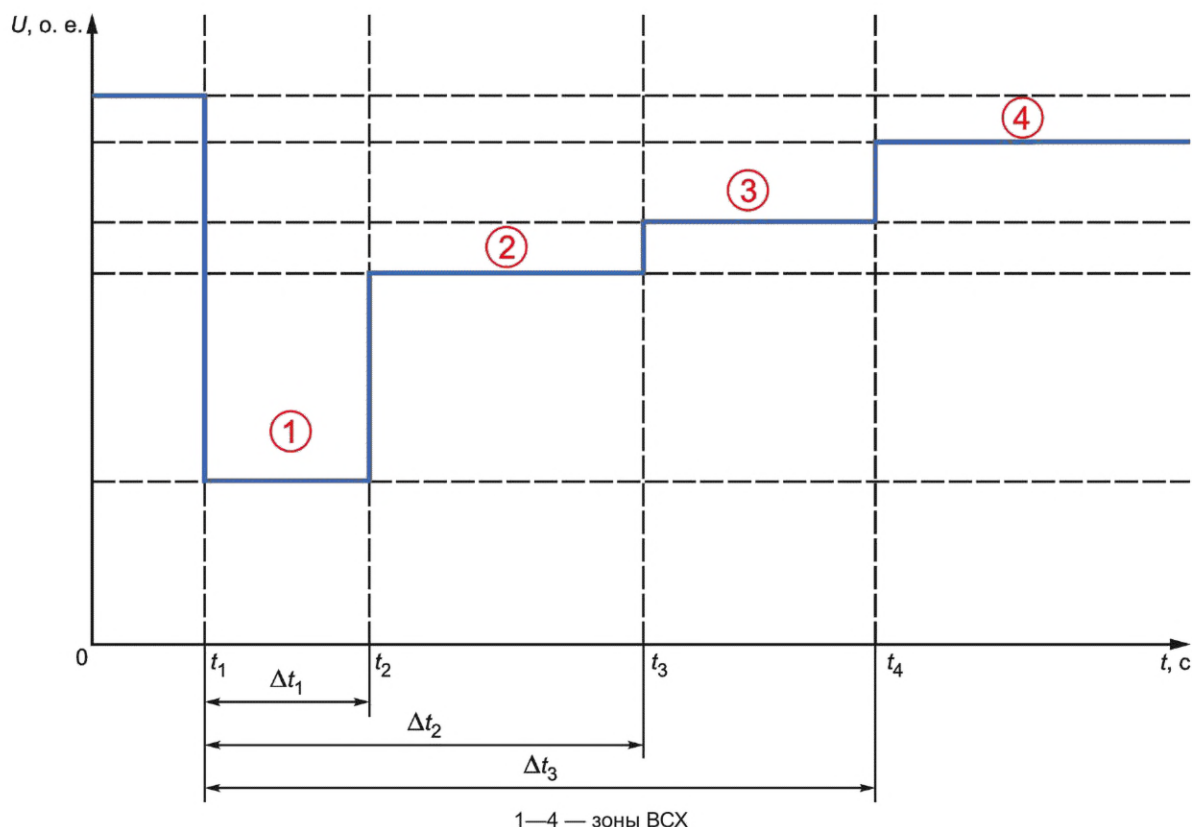
Рисунок А.1 — Общий вид ВСХ
