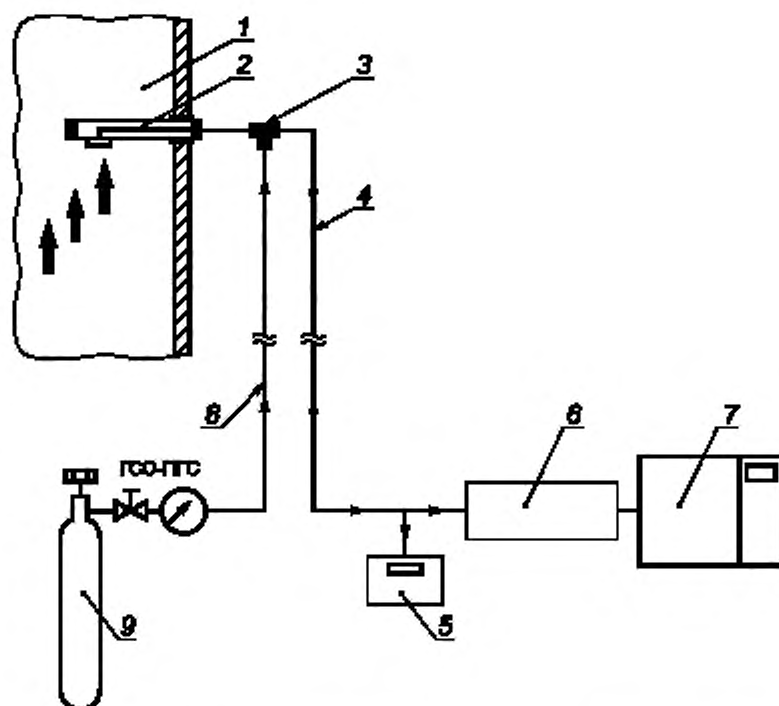
1 — газозод, 2 — зонд-пробоотборник АИС КВ; 3 — тройник-переключатель. 4 — трубопровод транспортировки пробы АИС КВ; 5 — аналитический блок для определения влажности (для АИС КВ с предварительным удалением паров воды при подготовке пробы). 6 — система подготовки пробы АИС КВ; 7 — газоналитический блок АИС КВ; 8 — линия для транспортировки ГСО-ПГС; 9 — баллон с газовой смесью ГСО-ПГС
