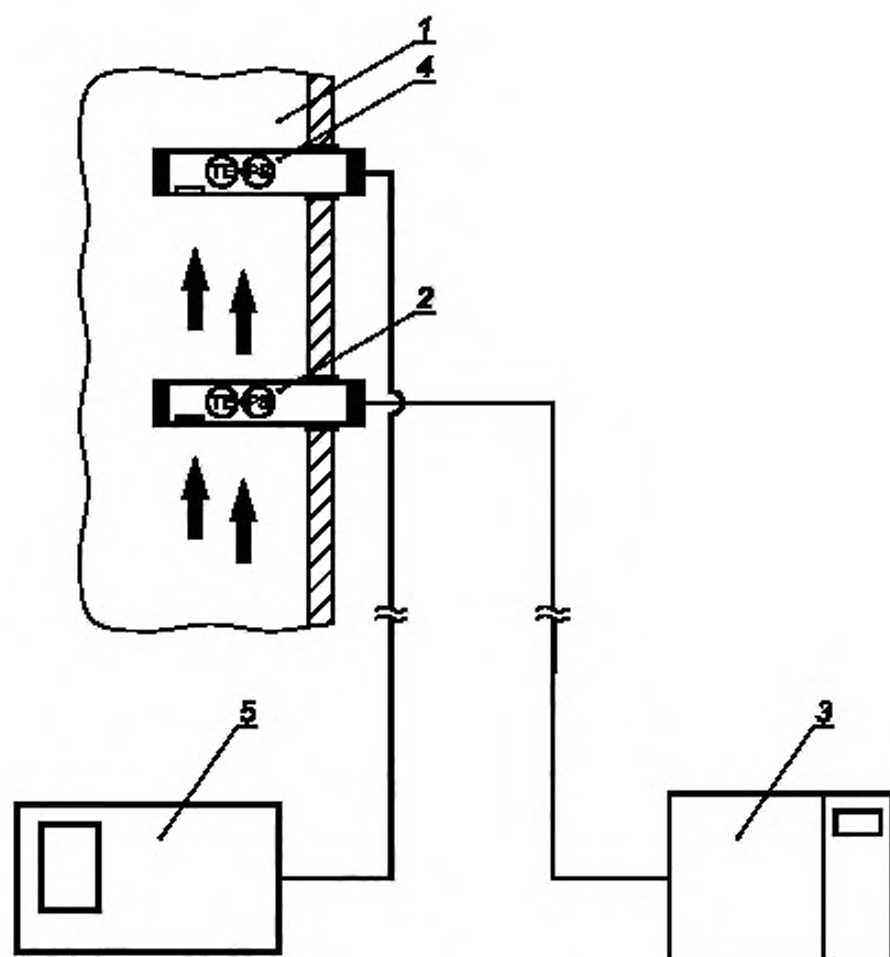
1 — газоход; 2 — зонд(ы) параметров газового потока АИС КВ с датчиками температуры и давления, 3 — аналитический блок параметров газового потока АИС КВ, 4 — зонд параметров газового потока эталонной системы с датчиками температуры и давления газового потока, 5 — эталонная система измерения параметров газового потока
