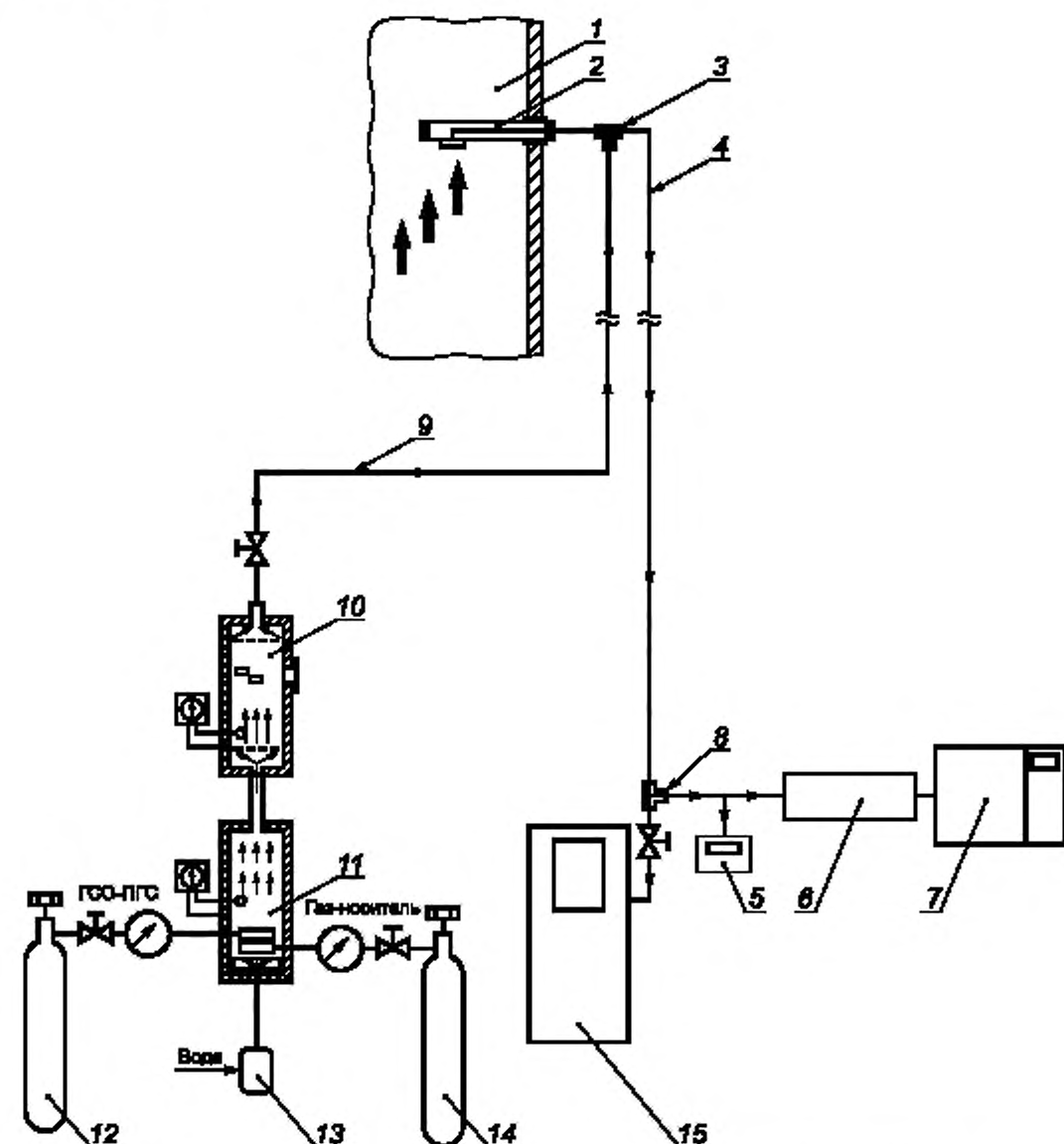
1 — газоход; 2 — зонд-пробоотборник АИС КВ; 3 — тройник-переключатель; 4 — трубопровод транспортировки пробы АИС КВ; 5 — аналитический блок для определения влажности (для АИС КВ с предварительным удалением паров воды при подготовке пробы); 6 — система подготовки пробы АИС КВ; 7 — газоаналитический блок АИС КВ; 8 — тройник; 9 — линия для транспортировки многокомпонентной увлажненной ГС на основе ГСО-ПГС; 10 — рабочая камера-смеситель; 11 — газовый генератор для получения многокомпонентной увлажненной ГС на основе ГСО-ПГС; 12 — баллон с многокомпонентной ГСО-ПГС; 13 — насос для подачи воды; 14 — баллон с газом-носителем — азотом; 15 — мобильный поверочный комплекс (с каналом определения влажности)
