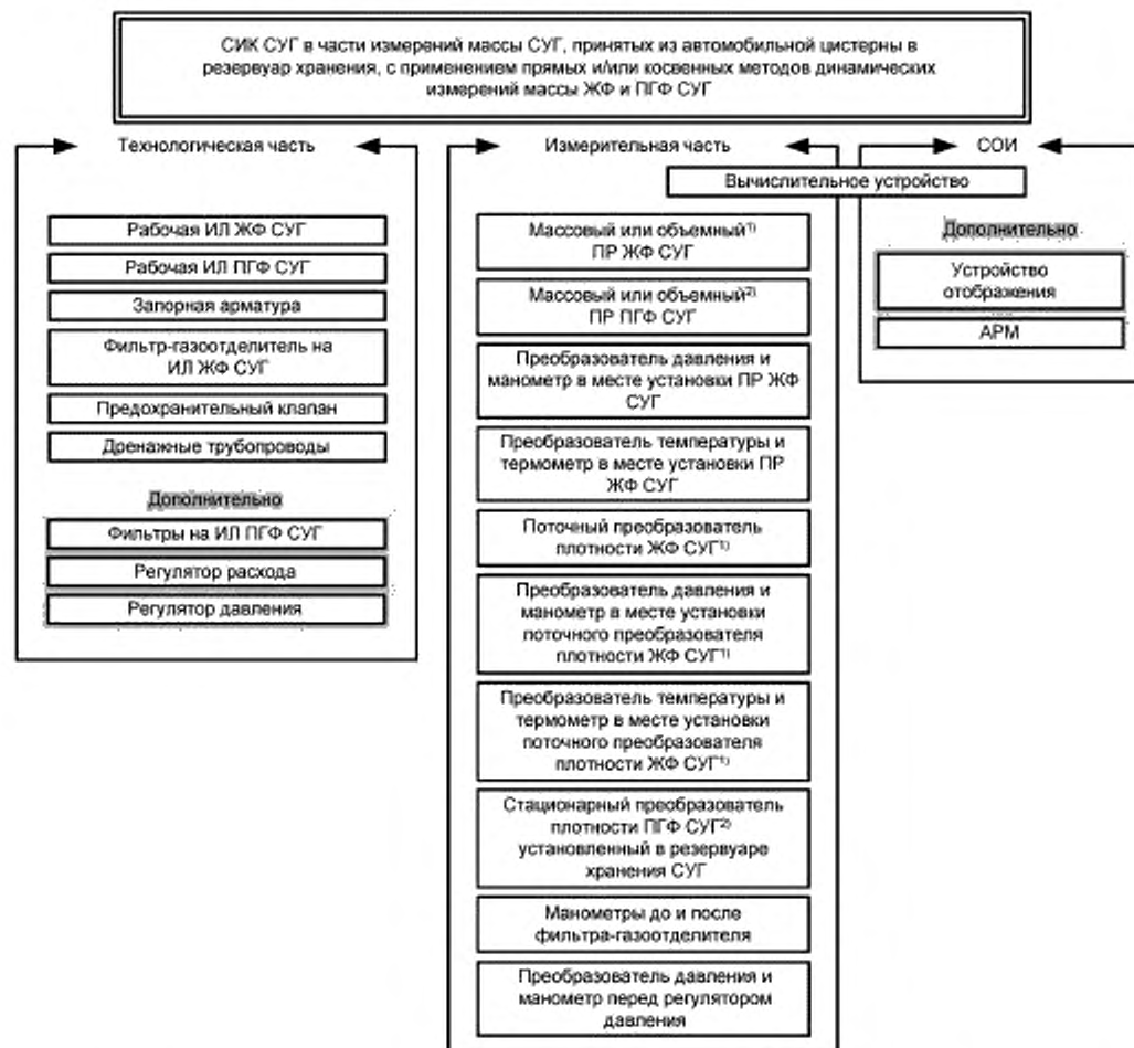
Рисунок В.1 — Структурная схема СИК СУГ в части измерений массы СУГ, принятых из автомобильной цистерны в резервуар хранения, с применением прямых и/или косвенных методов динамических измерений массы ЖФ и ПГФ СУГ
