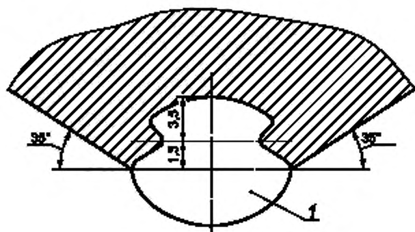
1 — контактный провод
