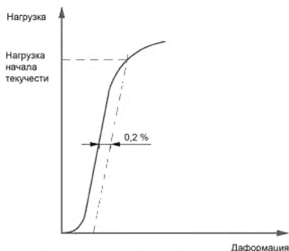
Рисунок В.3 — Определение нагрузки начала текучести
