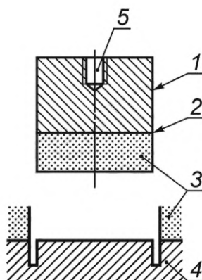
1 — металлическая пластинка; 2 — слой клея; 3 — слой затвердевшего раствора; 4 — основание; 5 — отверстие с внутренней резьбой по центру пластинки для крепления приспособления для отрыва образцов от основания
