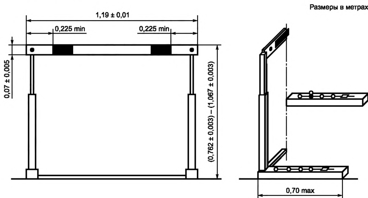
Рисунок 1 — Основные размеры элементов конструкции барьера для бега
