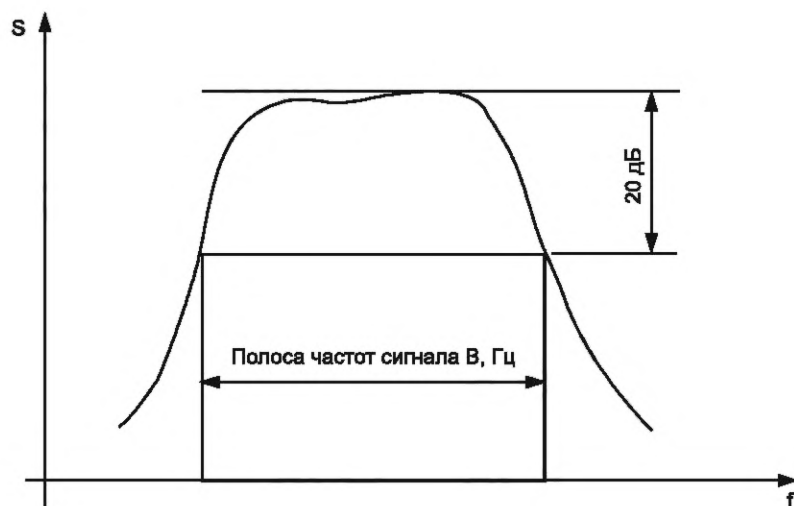
Рисунок 3 — Измерение полосы частот сигнала
