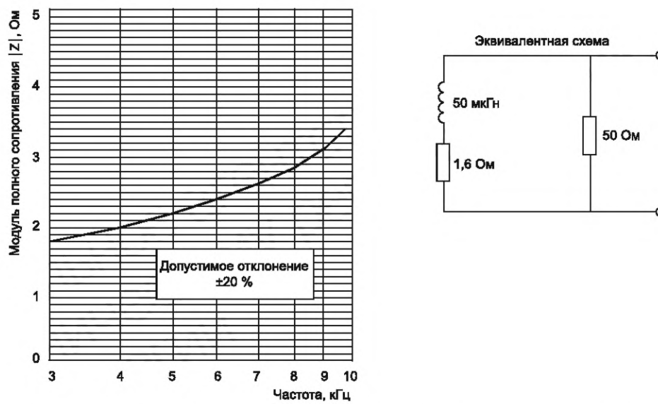
Рисунок 6 — Эквивалентная схема и модуль входного полного сопротивления эквивалента сети
