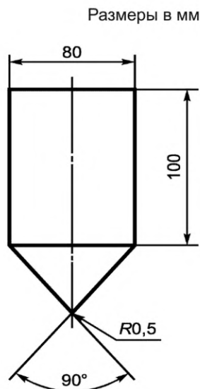
Рисунок 6 — Испытательный конус
