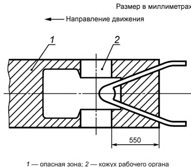
Рисунок 6 — Пределы опасной зоны в случае, когда устройство для запуска культиватора без реверсивной передачи
