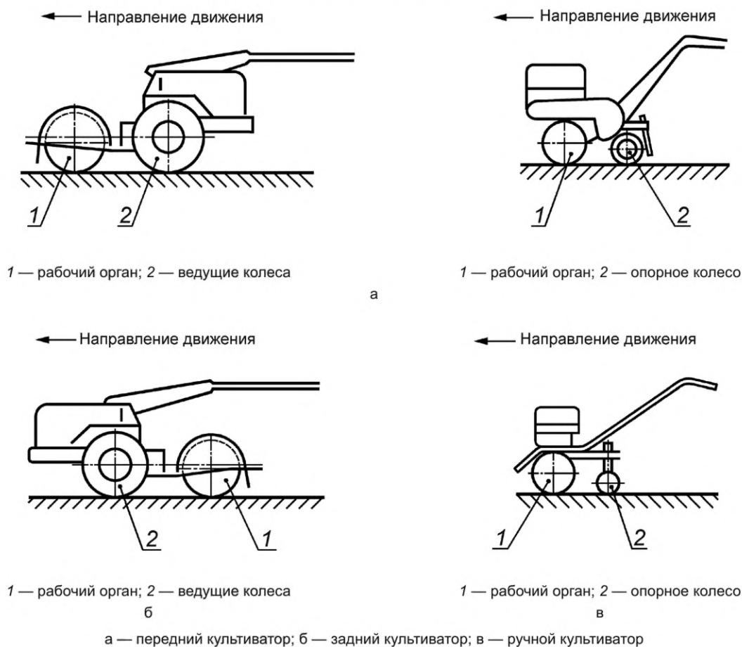
Рисунок 1 — Типы культиваторов
