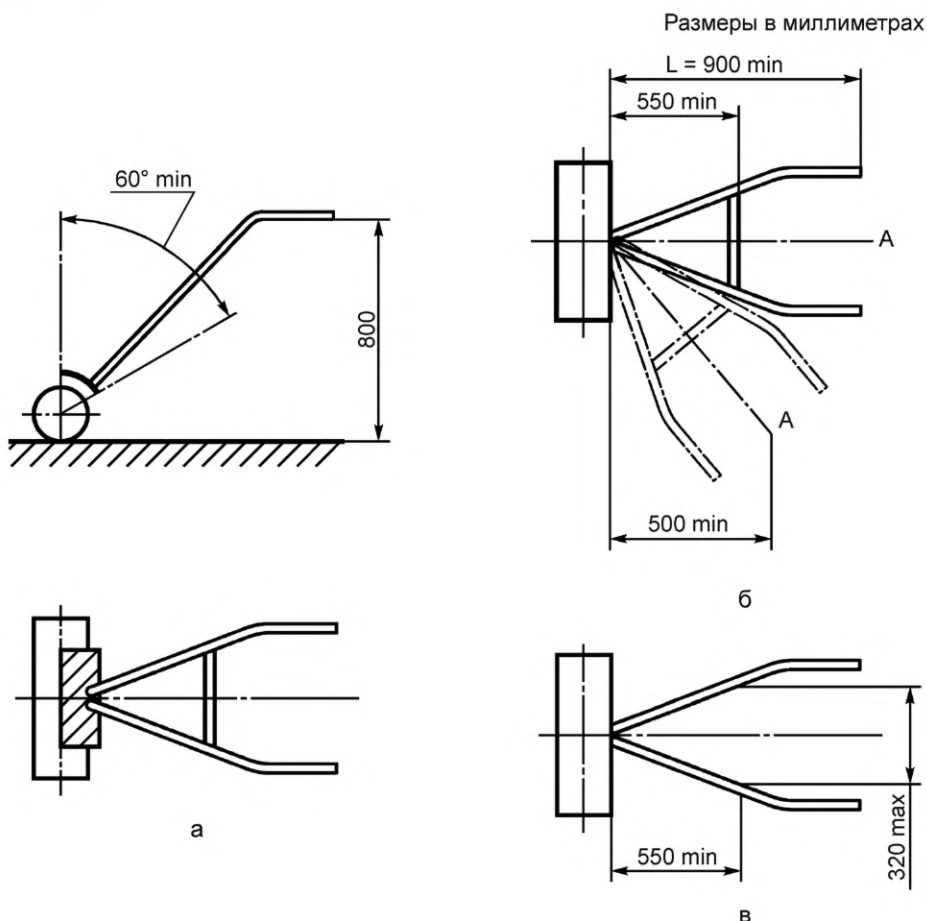
Рисунок 3 — Защита почвообрабатывающих органов переднего и ручного культиваторов
