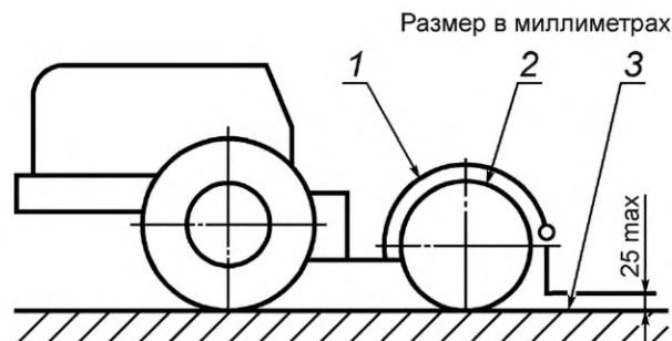
Рисунок 2 — Защита рабочего органа заднего культиватора
