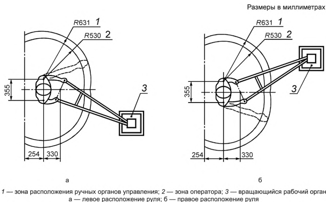
Рисунок 5 — Зона оператора, идущего рядом с культиватором
