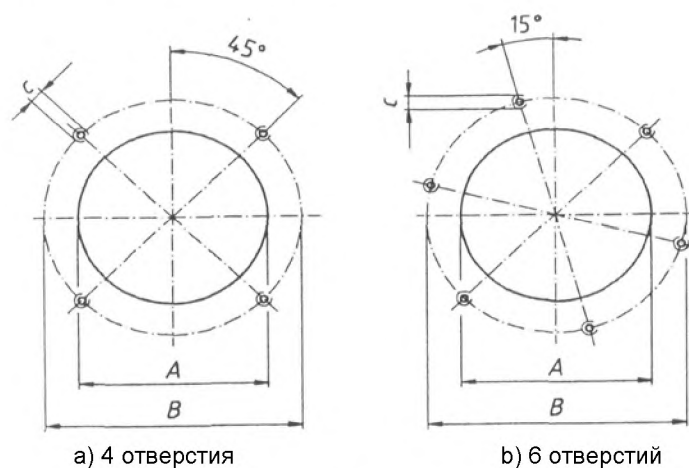
Рисунок 1 – Присоединительные размеры горелки
