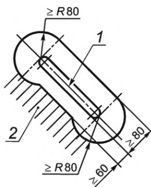
1 — рулевое колесо; 2 — неподвижные части машины
