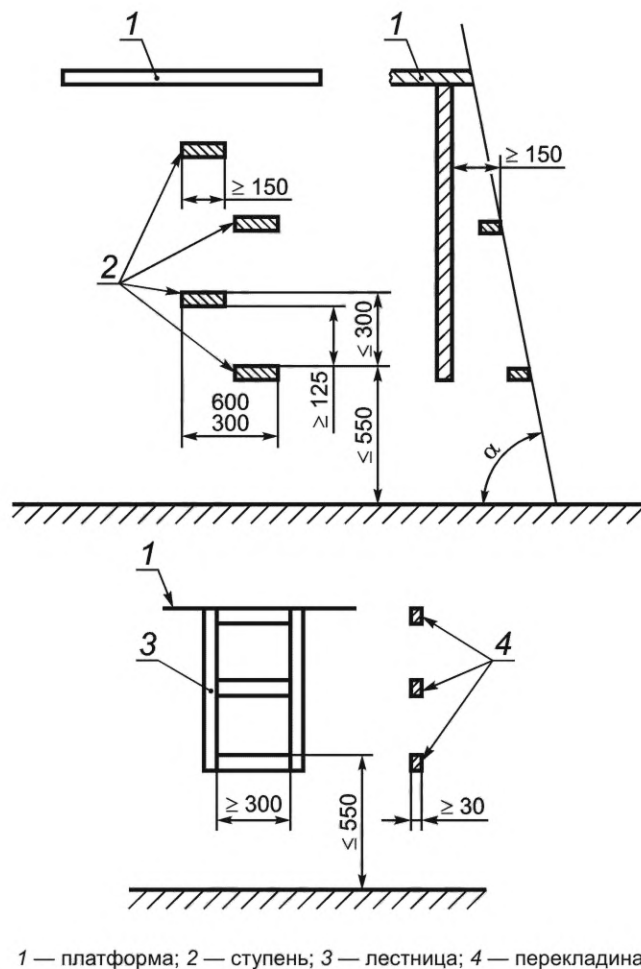
Рисунок 5 — Размеры средств доступа к другим местам, кроме рабочего места оператора
