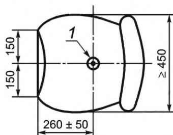
б) Координаты для измерения ширины сиденья
