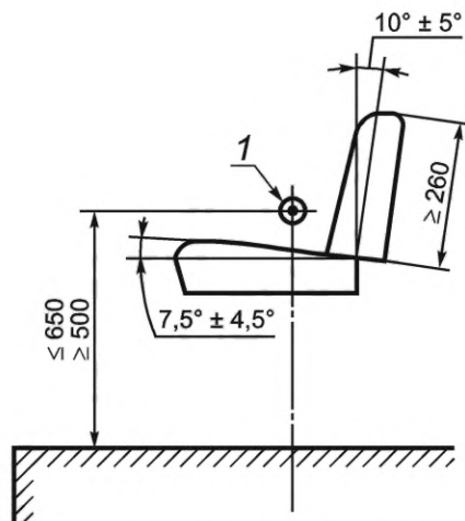
а) Диапазон регулировок сиденья
