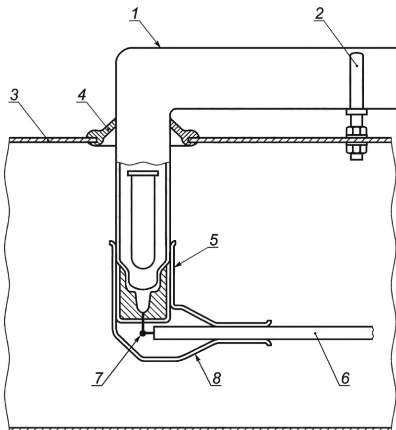
1 — газоразрядная лампа; 2 — опора для газоразрядной лампы в соответствии с требованиями 14.7.7; 3 — металлическая панель; 4 — уплотнение; 5 — пути утечки и воздушные зазоры в соответствии с требованиями 14.13; 6 — кабель; 7 — соединение в соответствии с требованиями 14.7.8; 8 — изоляционная втулка в соответствии с требованиями 14.7.1
