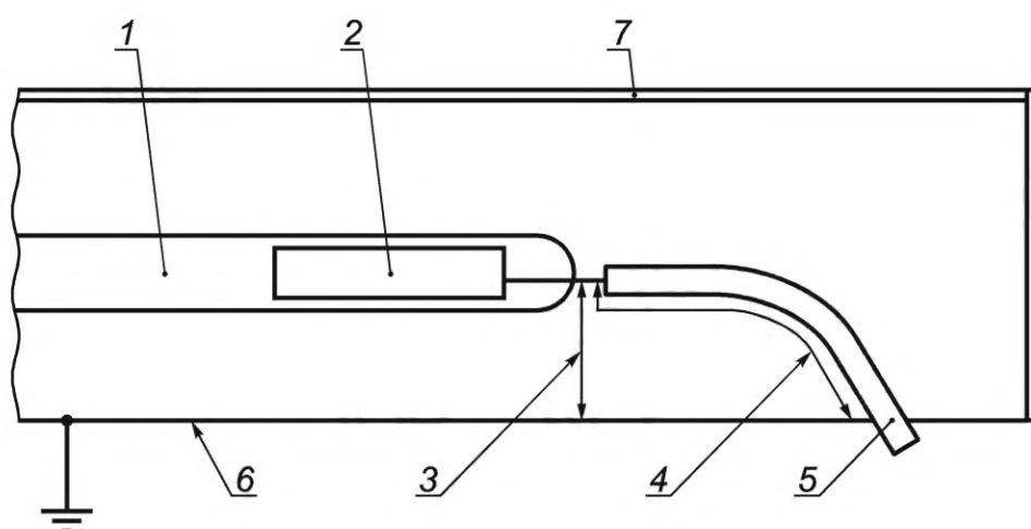
1 — лампа; 2 — электрод; 3 — воздушный зазор относительно земли; 4 — типичный путь утечки по поверхности изоляции; 5 — кабель; 6 — заземленная металлоконструкция; 7 — изоляционный материал
