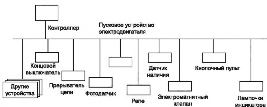
Рисунок 1 — Типовые интерфейсы DeviceNet между контроллерами и устройствами
