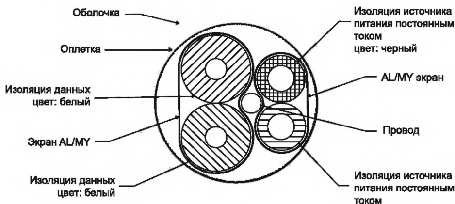
Рисунок 51 — Толстый кабель: физическая конфигурация
