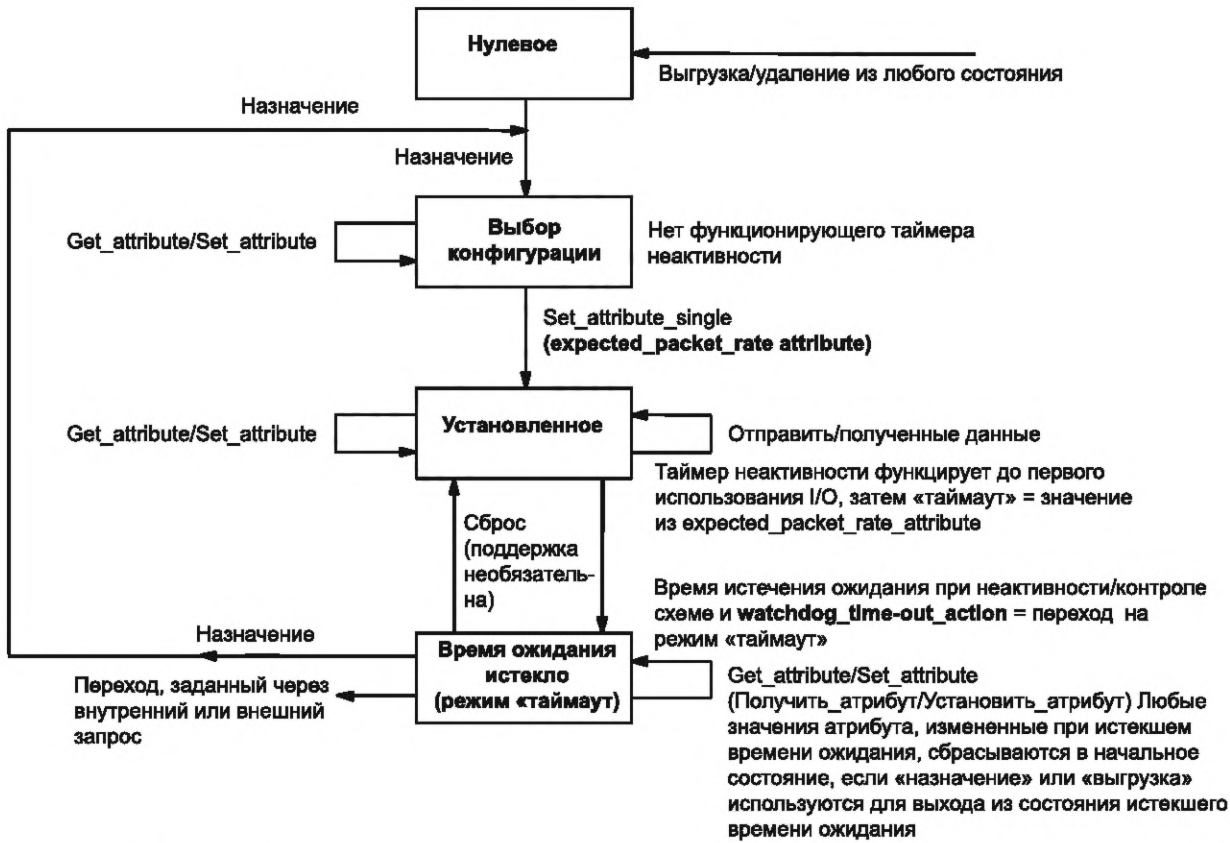
Рисунок 45 — Схема передачи состояния predetermined соединения I/O ведущего и ведомого устройств
