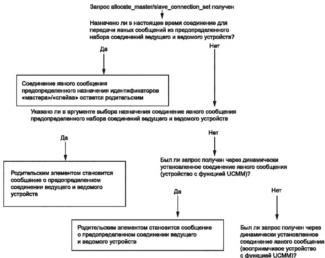
Рисунок 41 — Логическое описание соединения для передачи явных сообщений родительского элемента
