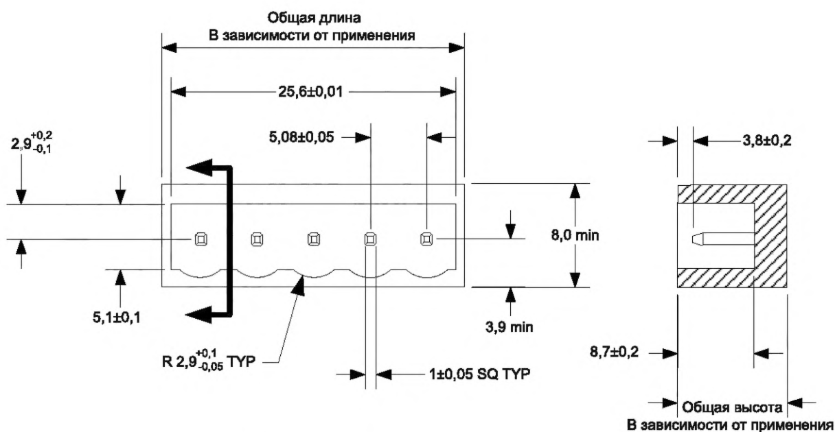
Рисунок 58 — Геометрия открытого разъема
