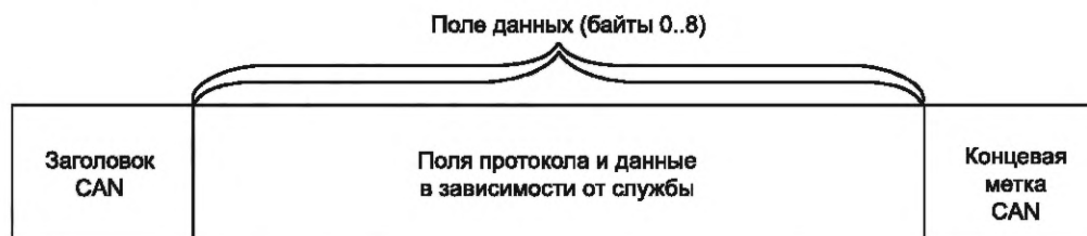
Рисунок 4 — Использование поля данных явного сообщения CAN
