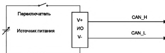
Рисунок 65 — Испытательная цепь включения питания
