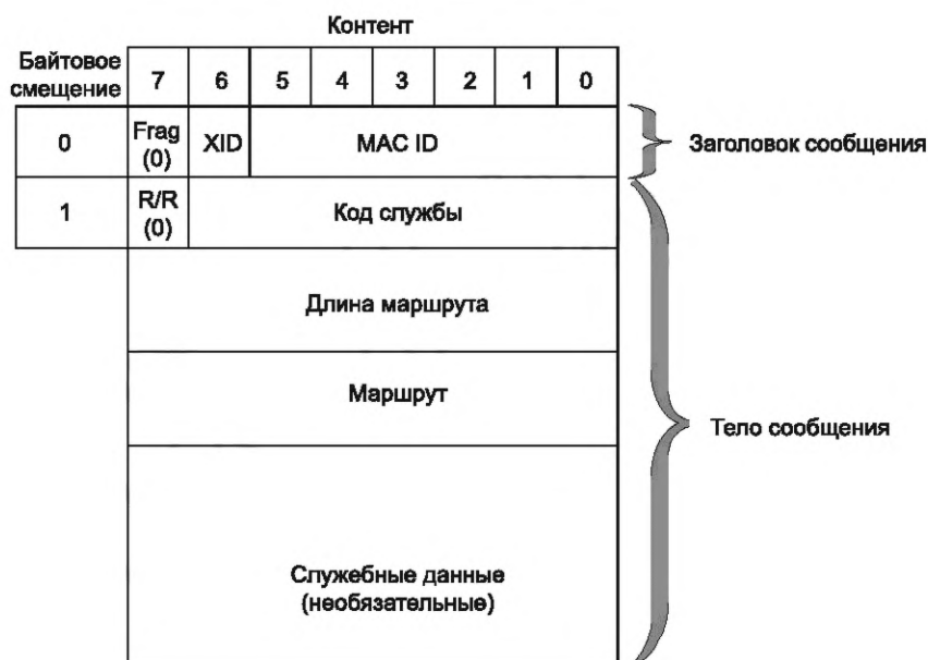
Рисунок 13 — Формат явного нефрагментированного сообщения-запроса, значение 4
