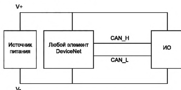
Рисунок 66 — Испытательная цепь для изменения полярности V+ и V-, а также прерывания подачи питания V-
