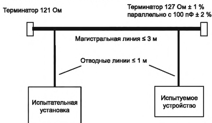
Рисунок 70 — Схема испытания временной выдержки
