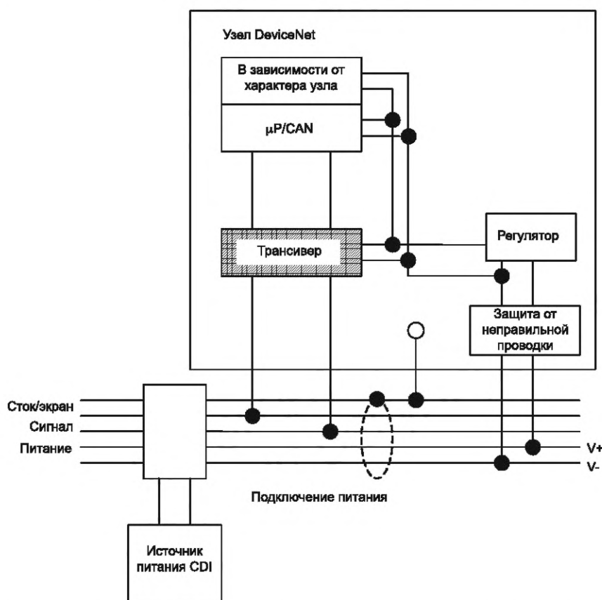
Рисунок 48 — Устройство, содержащее неизолированный физический уровень
