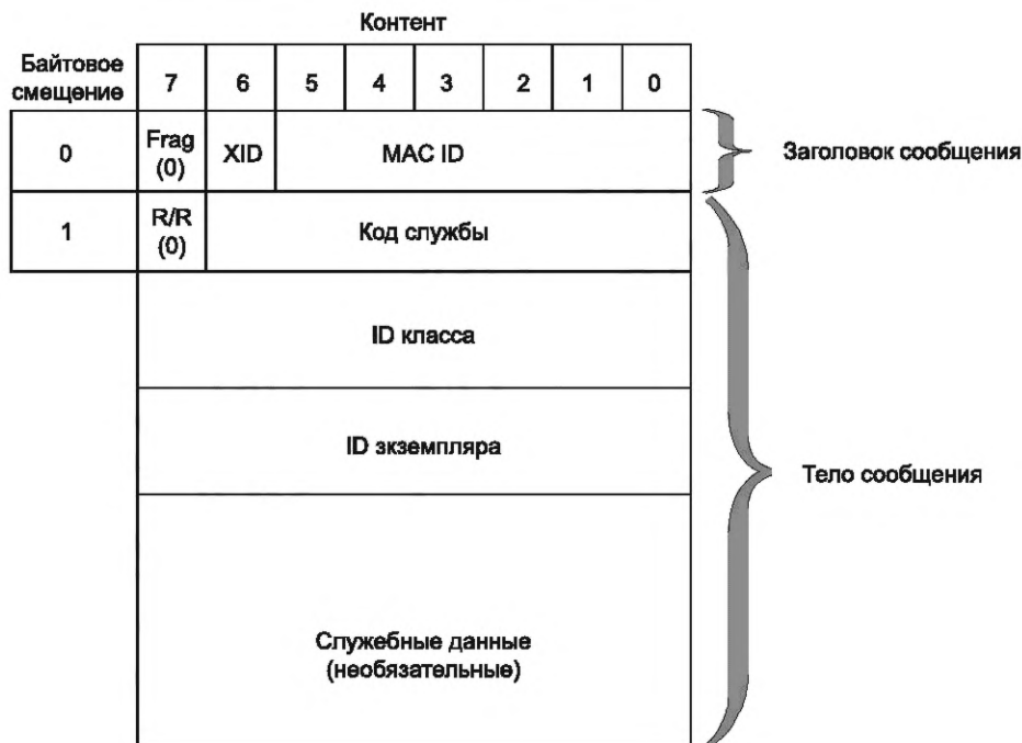
Рисунок 12 — Формат явного нефрагментированного сообщения-запроса, значения 0—3
