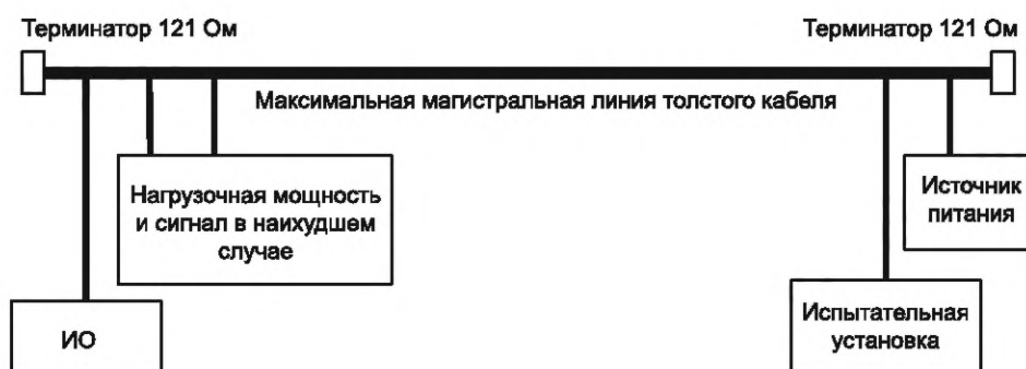
Рисунок 72 — Схема проведения испытания CDI
