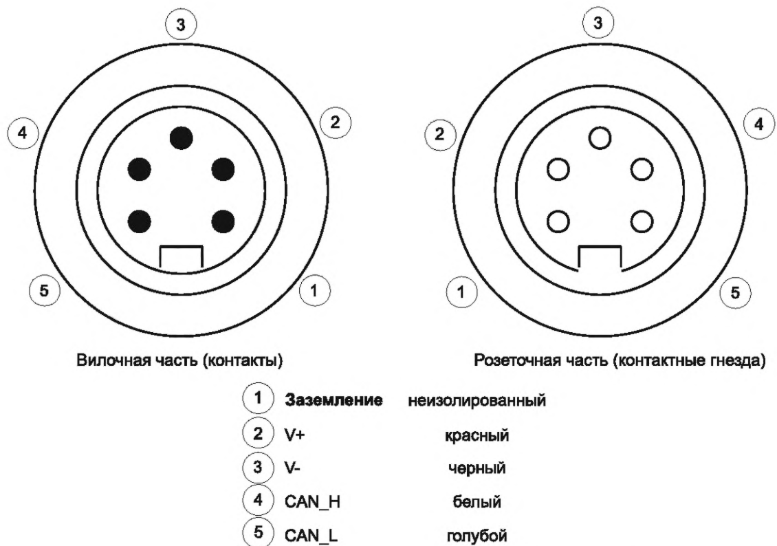
Рисунок 59 — Разводка контактов герметичного мини-разъема
