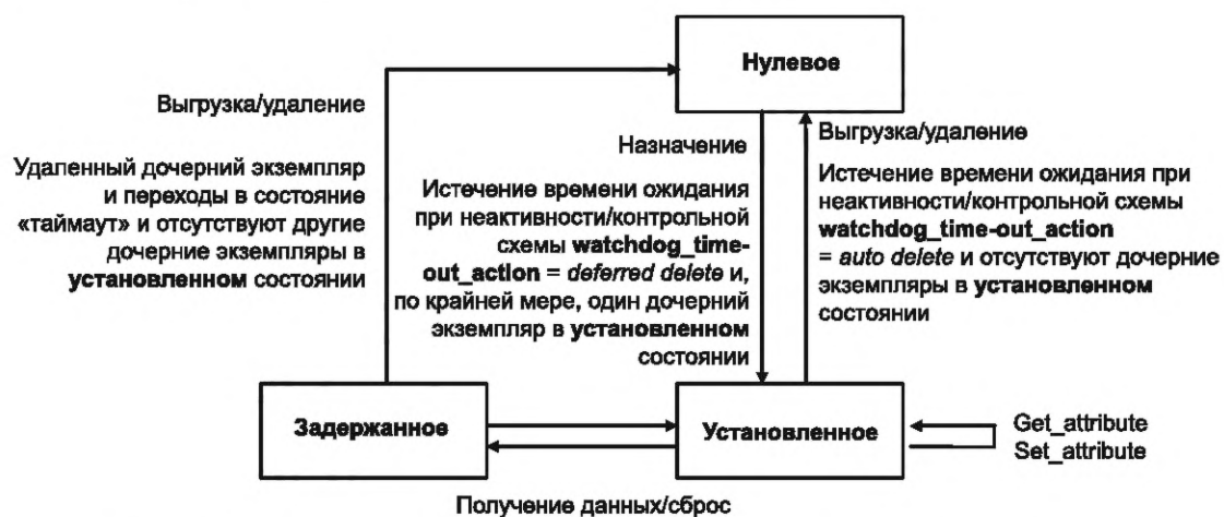
Рисунок 46 — Схема передачи состояния предопределенного соединения ведущего и ведомого устройства для передачи явных сообщений
