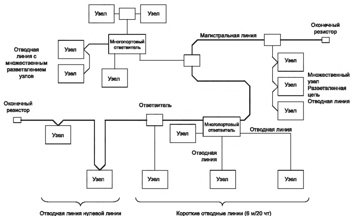
Рисунок 50 — Топология среды DeviceNet
