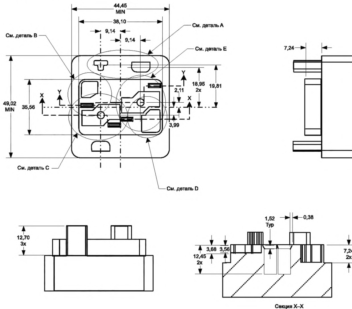
Рисунок 61 — Схема плоского разъема магистральной линии — разводка контактов
