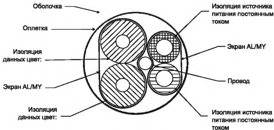
Рисунок 53 — Тонкий кабель: физическая конфигурация
