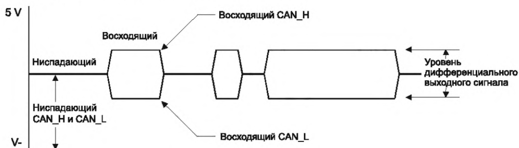
Рисунок 69 — Уровни передачи
