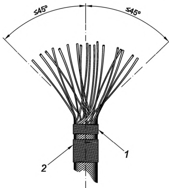
1 — постоянный бандаж; 2 — вспомогательный бандаж
