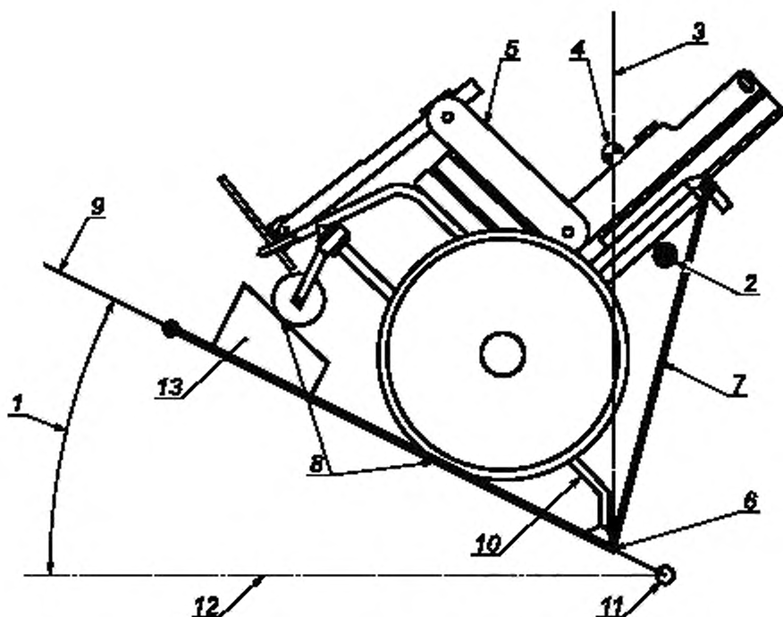
1 — угол наклона антипрокидывающих устройств; 2 — ограничитель наклона (см. 5.5); 3 — вертикаль; 4 — центр тяжести кресла-коляски с манекеном; 5 — испытательный манекен; 6 — ось опрокидывания; 7 — приспособление, препятствующее скольжению (см. 5.4); 8 — точки определения силы давления под колесами; 9 — испытательная платформа; 10 — заблокированное колесо или опорная стойка антипрокидывающих устройств; 11 — механизм, регулирующий наклон испытательной платформы; 12 — горизонталь; 13 — клинообразная подкладка
