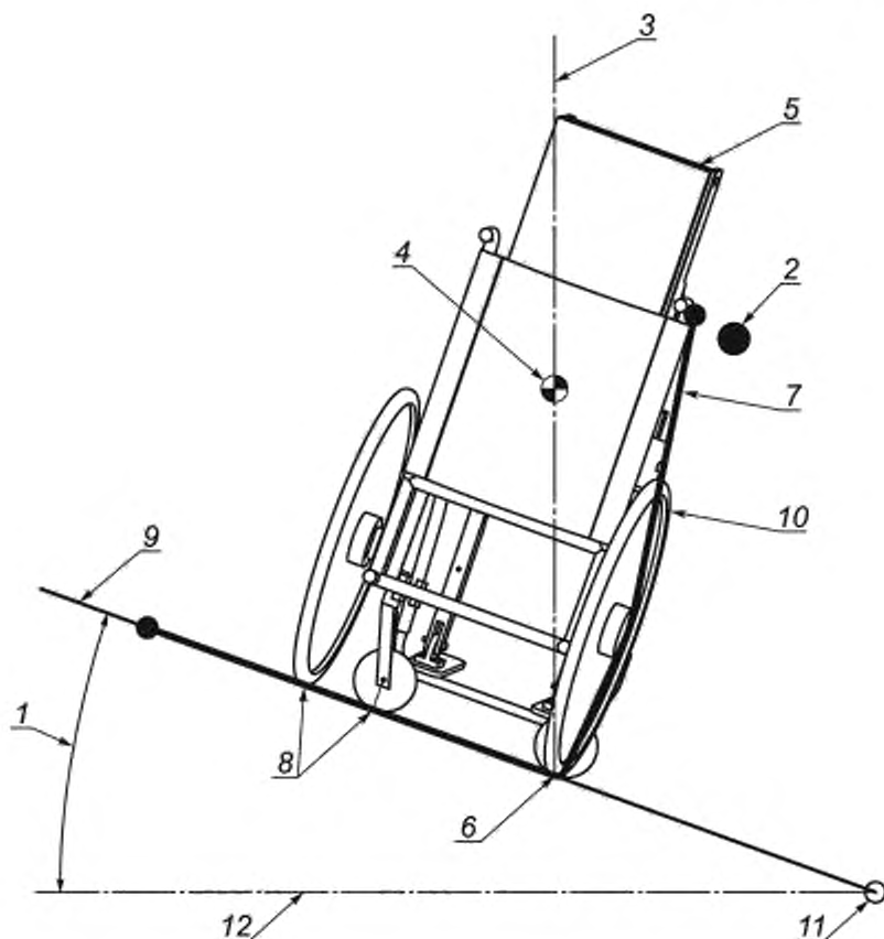
1 — угол наклона кресла-коляски; 2 — ограничитель наклона; 3 — вертикаль; 4 — центр тяжести кресла-коляски с манекеном; 5 — испытательный манекен; 6 — ось опрокидывания; 7 — приспособление, препятствующее скольжению (см. 5.4); 8 — точки определения силы давления под колесами; 9 — испытательная платформа; 10 — заблокированное или незаблокированное колесо; 11 — механизм, регулирующий наклон испытательной платформы; 12 — горизонталь
