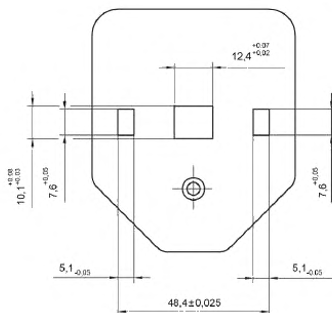
Рисунок А.3 — Крышка
