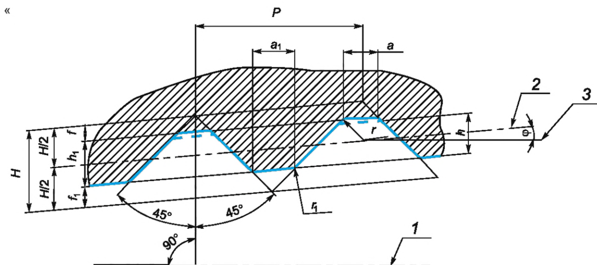
а — профиль резьбы муфтового конца
