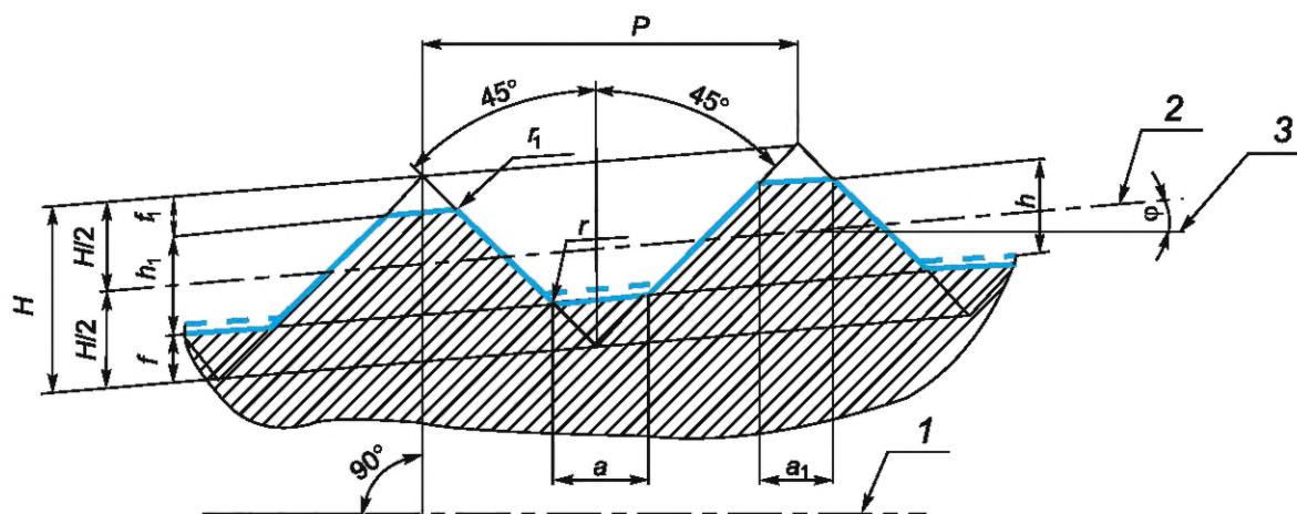
б — профиль резьбы nippleного конца
