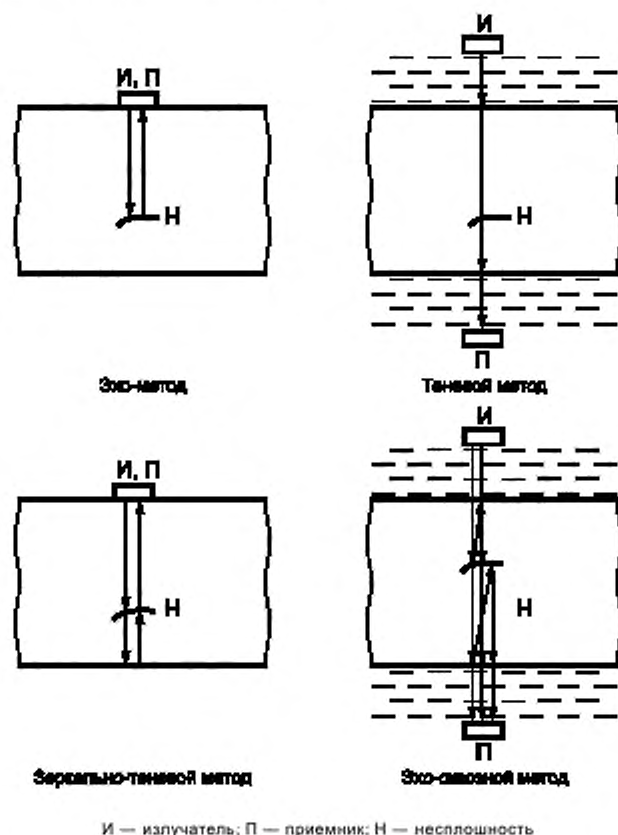
Рисунок 2 — Методы УЗК продольными волнами
