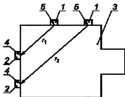
1 — излучатель; 2 — приемник; 3 — ОК; 4, 5 — точки ввода
