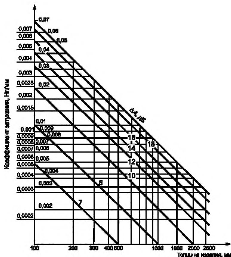
Рисунок А.2 — Номограмма для определения коэффициента затухания
