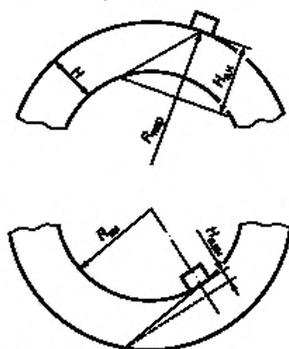
Рисунок 6 — Эквивалентная толщина ОК цилиндрической формы
