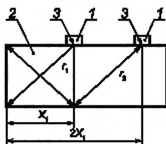
1 — ПЭП; 2 — изделие; 3 — точка ввода
