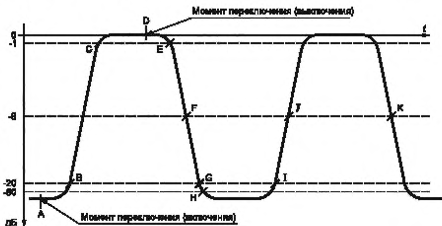
Рисунок 1 — График изменения огибающей испытательного сигнала
