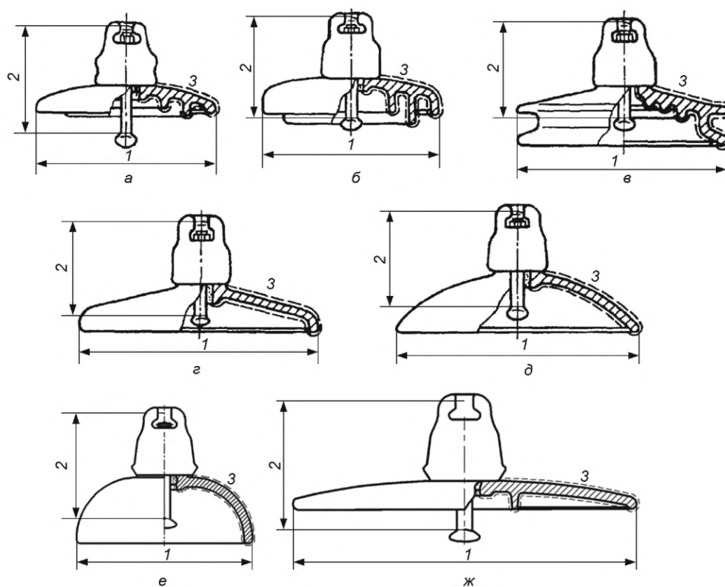
а — стандартная (со слаборазвитой поверхностью изоляционной детали); б — с увеличенным вылетом ребра (В); в — двурылая (Д); г — коническая (К); д — сферическая (С); е — колоколообразная (КЛ); ж — аэродинамическая (А или АД, или ВА); 1 — диаметр; 2 — строительная высота; 3 — длина пути утечки
