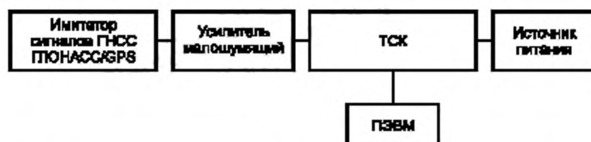
Рисунок А.1 — Схема испытательного стенда для проверки работоспособности ТСК
