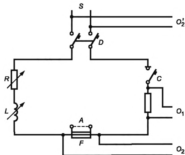
A — съемная перемычка применяемая при калибровке испытательной цепи; C — замыкающий выключатель; D — автоматический выключатель или другой защитный аппарат для защиты от пробоя; F — испытуемый плавкий предохранитель; L — настраиваемая катушка индуктивности; O 1 — измеритель для записи тока; O 2 — измеритель для записи напряжения при испытании; O' 2 — измеритель для записи напряжения при настройке; R — настраиваемое активное сопротивление; S — источник питания
