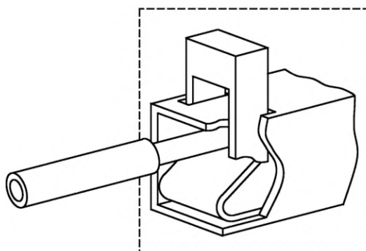
Безвинтовой вывод с промежуточным приводным элементом
