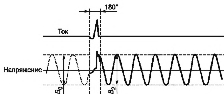
Рисунок 6b — Осциллограмма соответствующая операции отключению тока при которой дуга образуется после угла 180^\circ от момента включения
