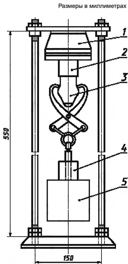
Рисунок 115 — Установка для проверки усилия расчленения
