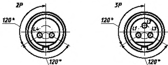
Расположение контактных гнезд
