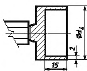
Калибр В для проверки диаметра d_4
