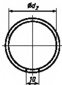
Калибр А для проверки диаметра d_2
