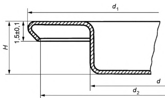
Рисунок А.6 — Пробка
