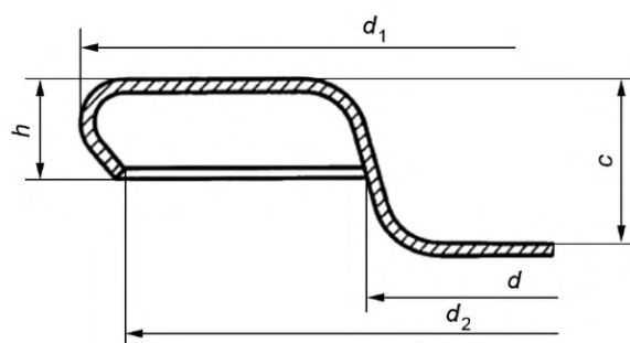
Рисунок А.7— Крышка
