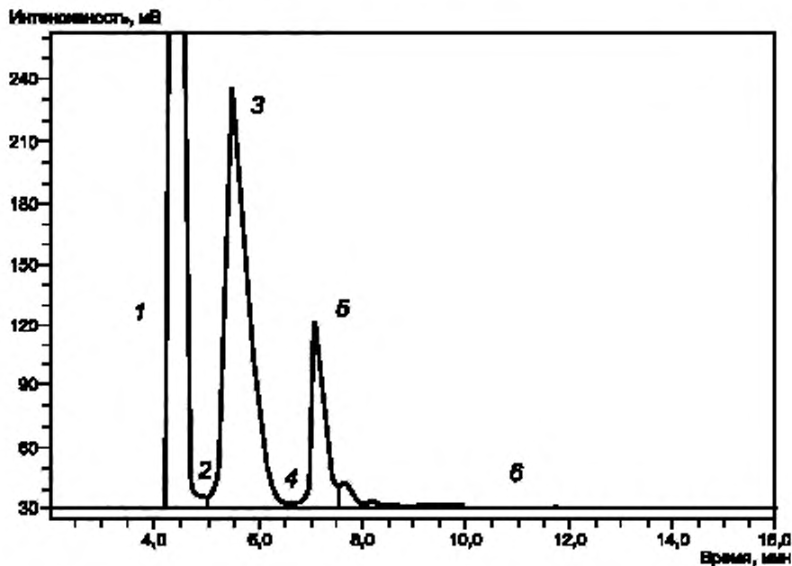
1 — неароматические углеводороды, 2 — начало интегрирования МАН, 3 — моноароматические углеводороды, 4 — конец интегрирования МАН/начало интегрирования ДАН; 5 — диароматические углеводороды, 6 — конец интегрирования ДАН
