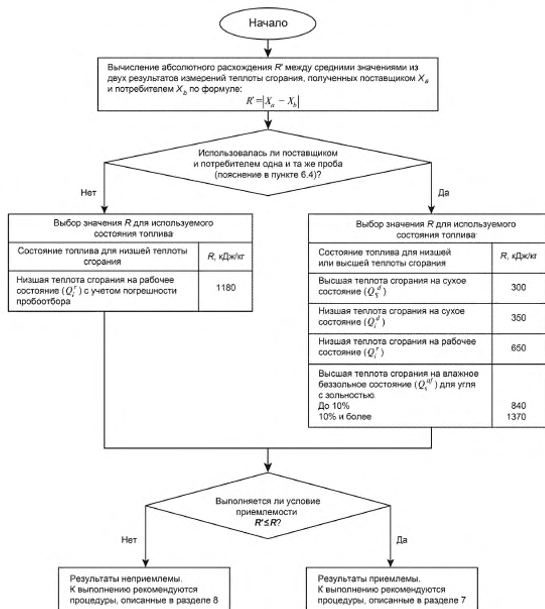
Рисунок 1 — Блок-схема проверки приемлемости результатов измерений
