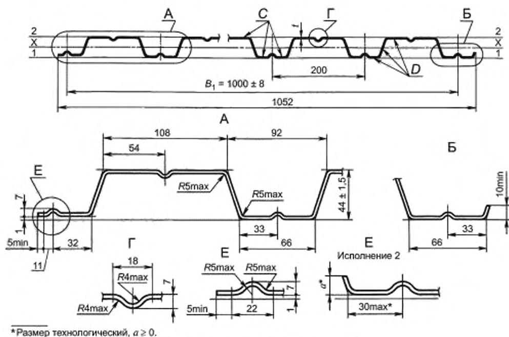
Рисунок Б.7 — Профили типа НС высотой 44 мм
