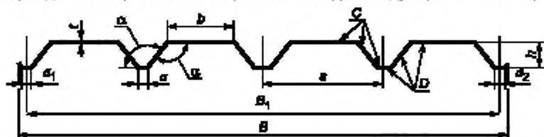
В 1 — монтажная ширина профиля; В — общая ширина; h — высота профиля; t — толщина профиля; s — шаг гофров; a и b — ширина полков профиля (в ряде случаев a = b); a 1 и a 2 — ширина крайних полков гофров профиля, C — наружная (лицевая) сторона профиля; D — обратная сторона профиля
