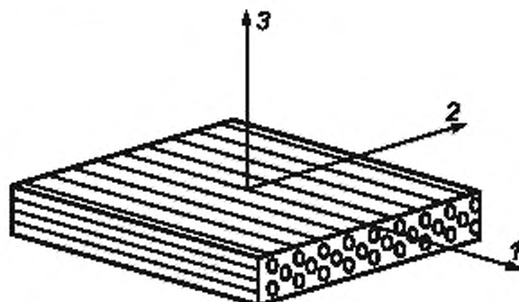
Рисунок 1 — Элемент пластины из композитного материала, армированного однонаправленным волокном, с указанием осей симметрии
