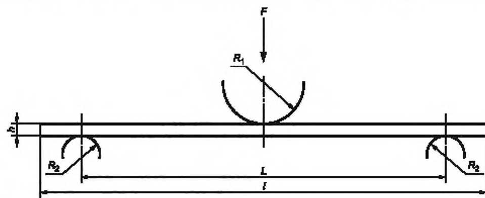
h — толщина образца, R_1 — радиус закругления пуансона, R_2 — радиус закругления краев опор, L — пролет между опорами, l — длина образца
