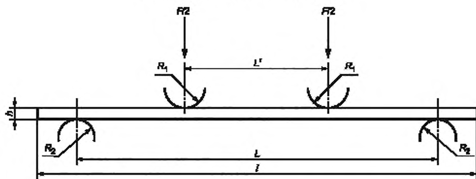
h — толщина образца, R_1 — радиус закругления пуансона, R_2 — радиус закругления краев опор, L — пролет между опорами, L' — пролет между верхними опорами, l — длина образца
