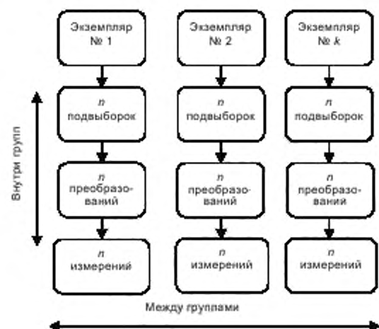
Рисунок 1 — План исследования однородности между экземплярами [22]
