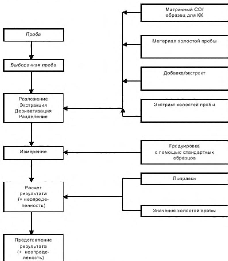
Рисунок 5 — Часть измерительной цепи
