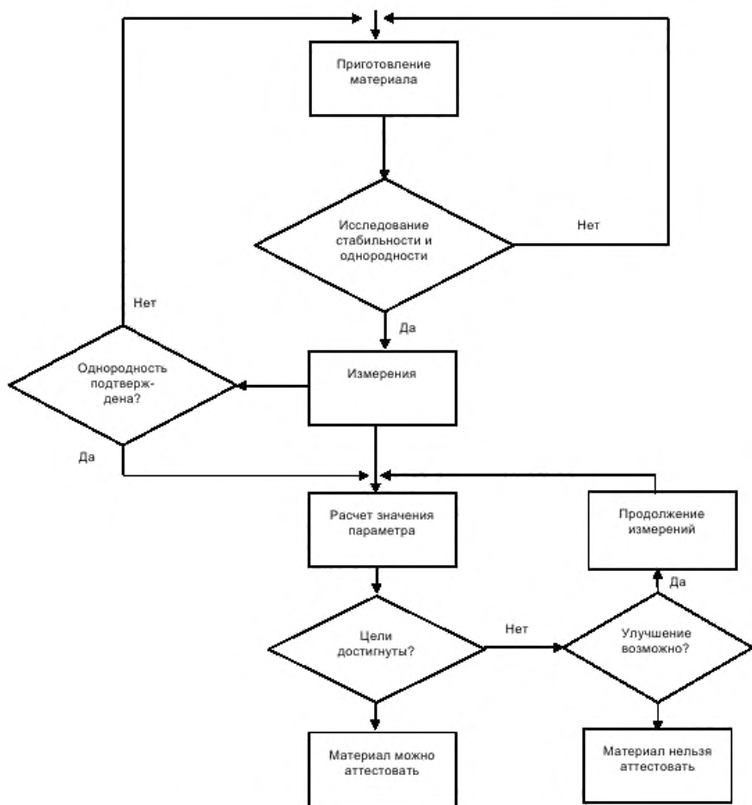
Рисунок 6 — План эксперимента при проведении измерений
