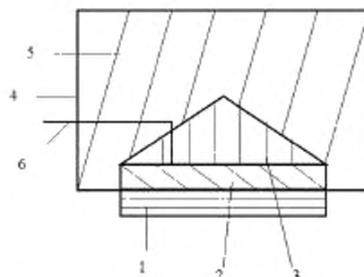
Рисунок Б.2 — Конструкция пьезопреобразователя поперечных волн
