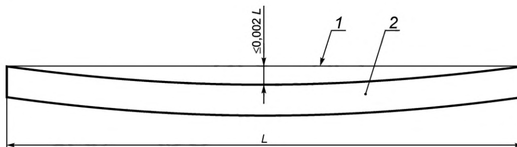
Рисунок 1 — Измерение общей прямолинейности
