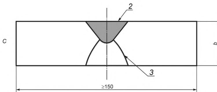
С — После ремонтной сварки — Вид в разрезе
