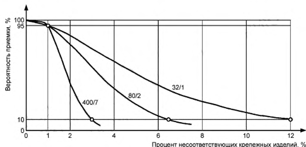
Пример — AQL = 1, планы выборочного контроля 32/1, 80/2 и 400/7.
