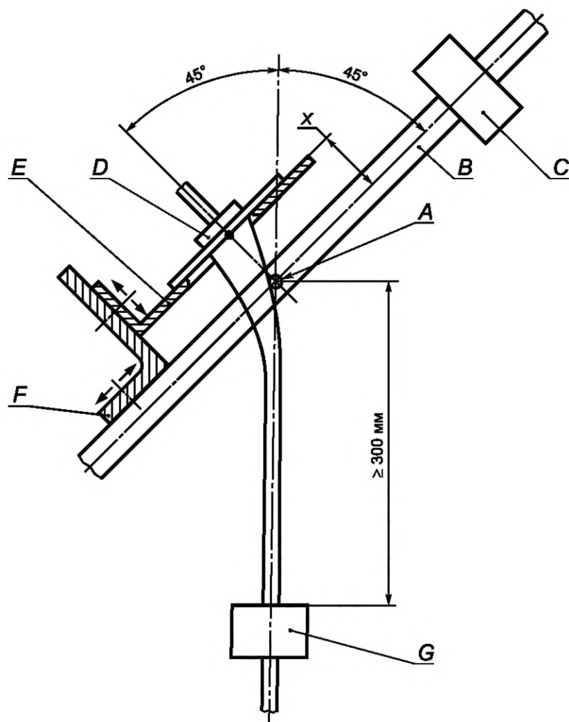
A — ось качания; B — качающийся элемент; C — противовес; D — образец; E — регулируемая несущая пластина; F — регулируемый держатель; G — груз
