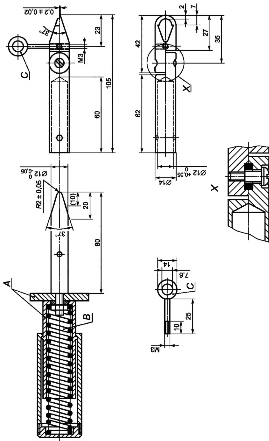
А — изоляционный материал; В — пружина, обеспечивающая толкающую силу на испытательном пружинном пальце по 22.11; С — петля
