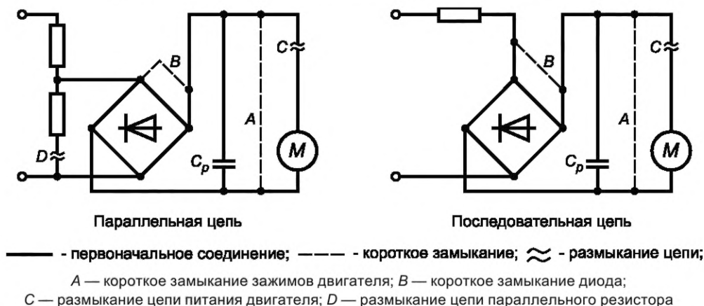
Рисунок I.1 — Имитация условий неисправности
