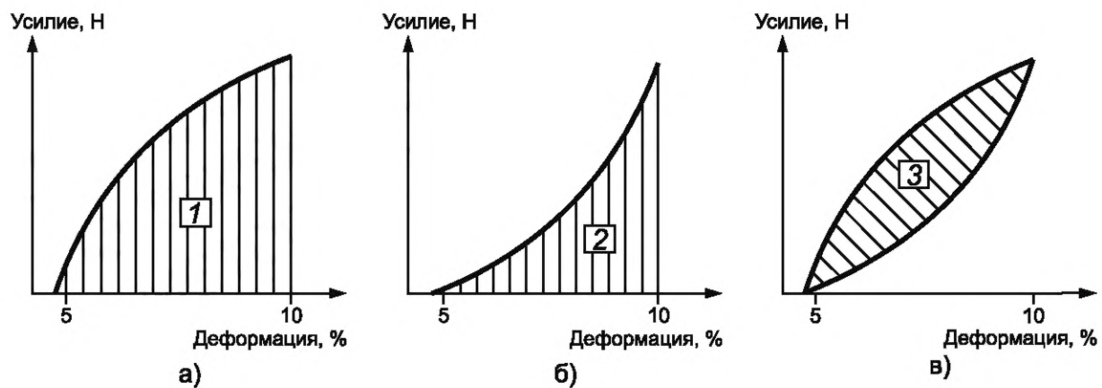
Рисунок С.3 — Работа цикла нагружение/разгрузка
