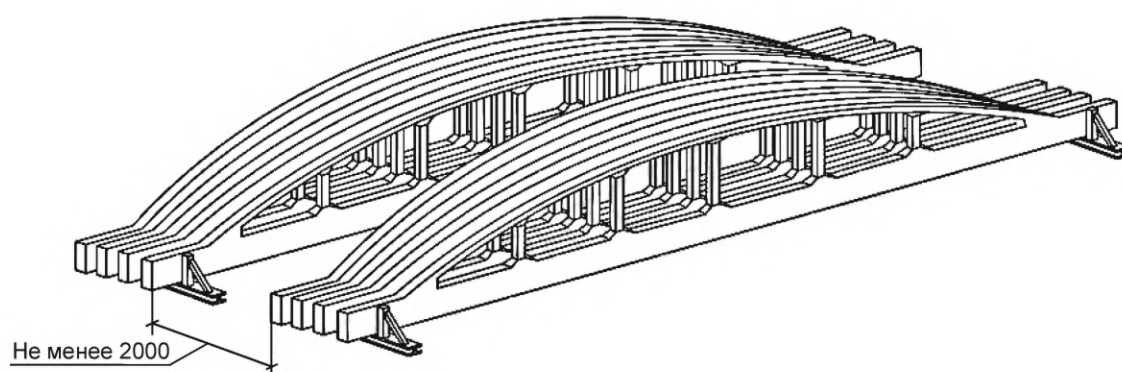
Рисунок 1 — Складирование ферм
