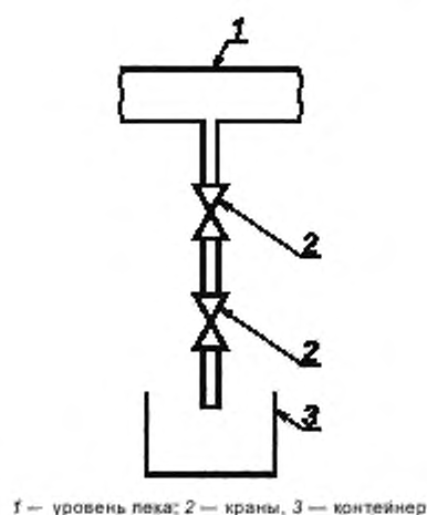
Рисунок 10 — Пробоотборник в виде трубопровода с двойным краном
