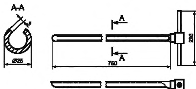
Рисунок 3 — Пробоотборник закрытого типа — типичные размеры
