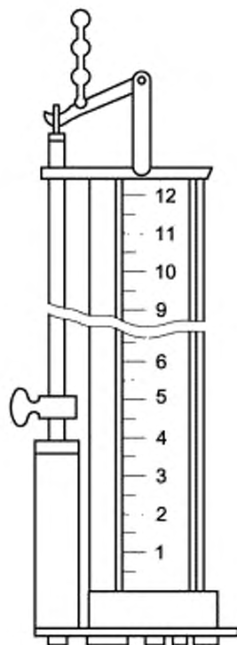
Рисунок 7 — Пробоотборник проточного типа (желонка)
