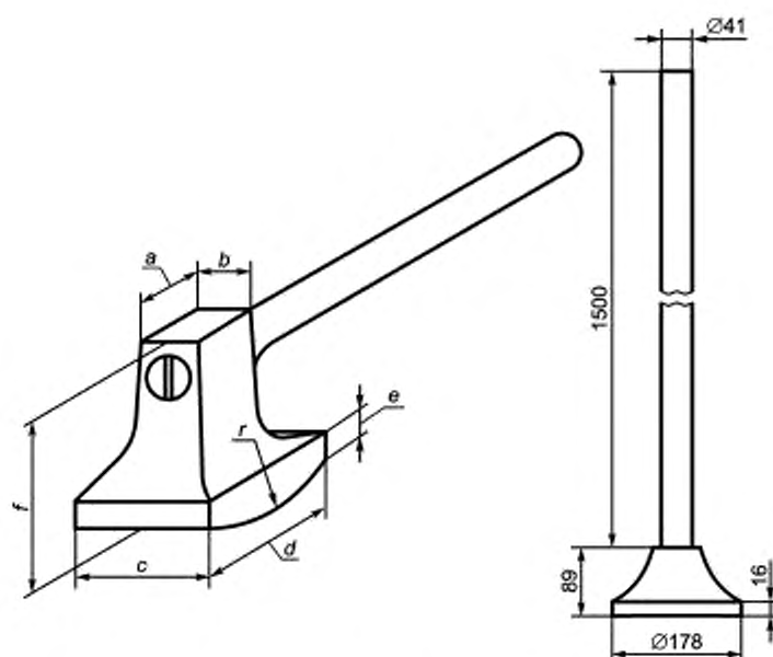
Рисунок 4 — Типичный молоток для дробления крупных частиц (кусков)
