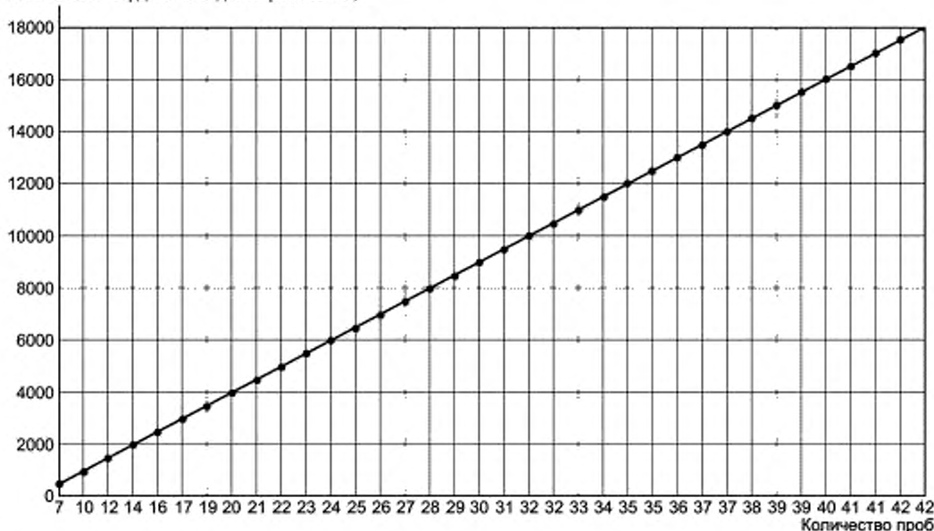
Рисунок 1 — Количество проб твердого пека в зависимости от количества пека, качество которого определяют
