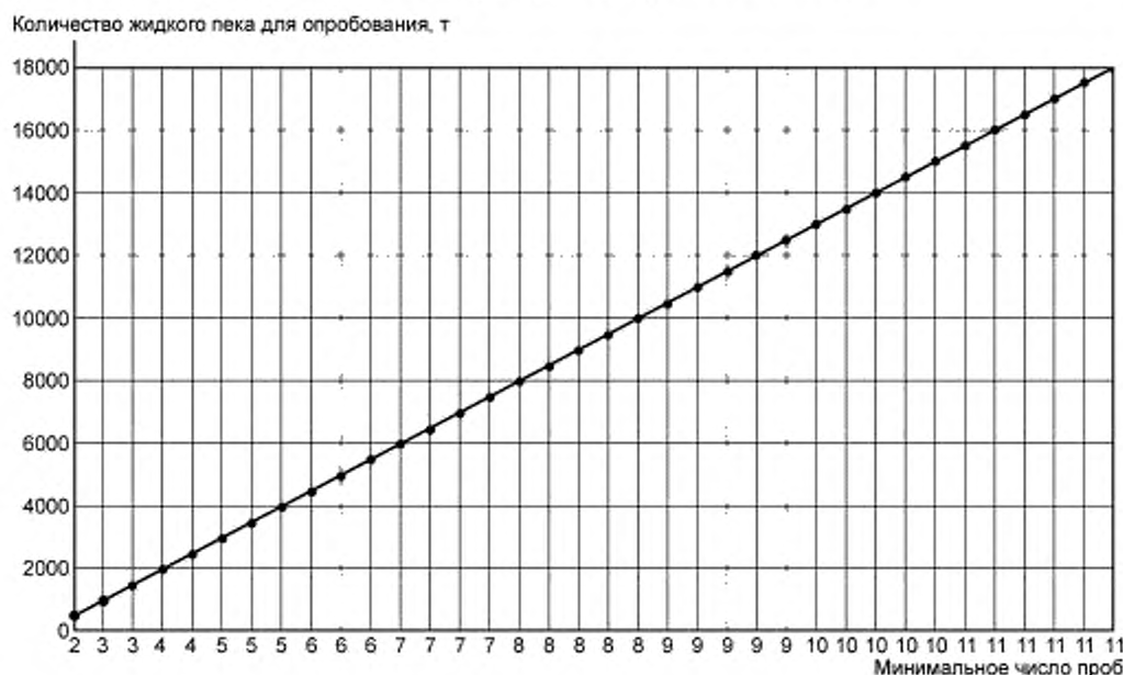
Рисунок 6 — Количество проб жидкого пека в зависимости от количества пека, качество которого определяют
