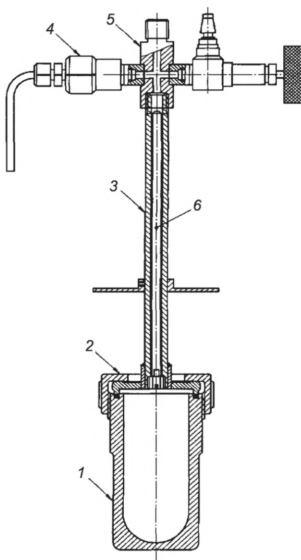
Рисунок 1, лист 1 — Бомба с мембранным предохранительным устройством для определения окислительной стабильности бензина
