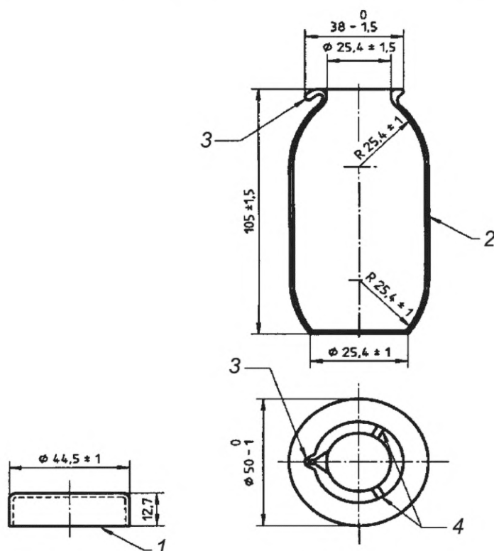
1 — крышка (стеклянная или фарфоровая); 2 — контейнер для пробы (стеклянный) толщиной стенки ( 2,0 \pm 0,5 ) мм; 3 — слив; 4 — две прорези или углубления
