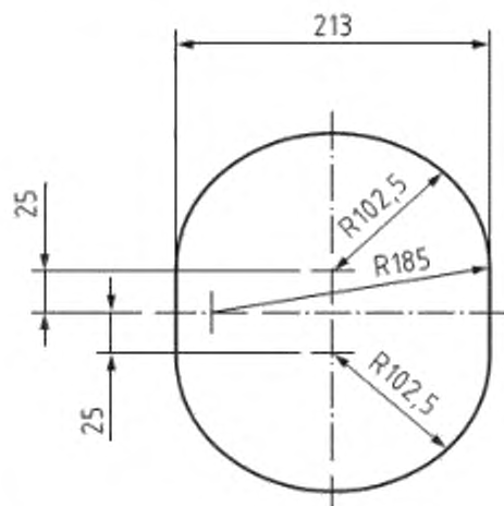
Рисунок 2 — Размеры отверстия в нижней части термокамеры
