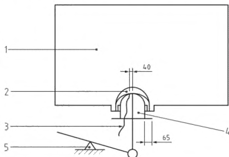
1 – термокамера; 2 – испытуемый образец; 3 – термопара; 4 – термомакет; 5 – подъемное устройство
